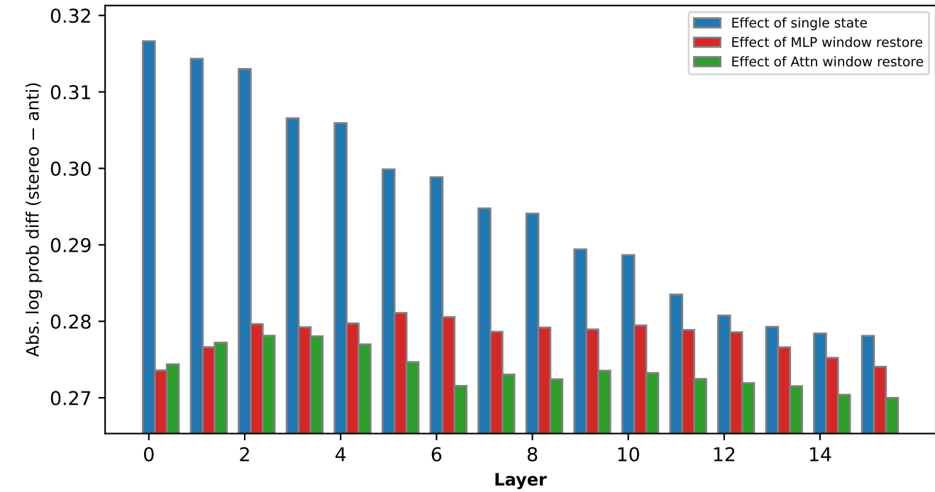
s2-24B
