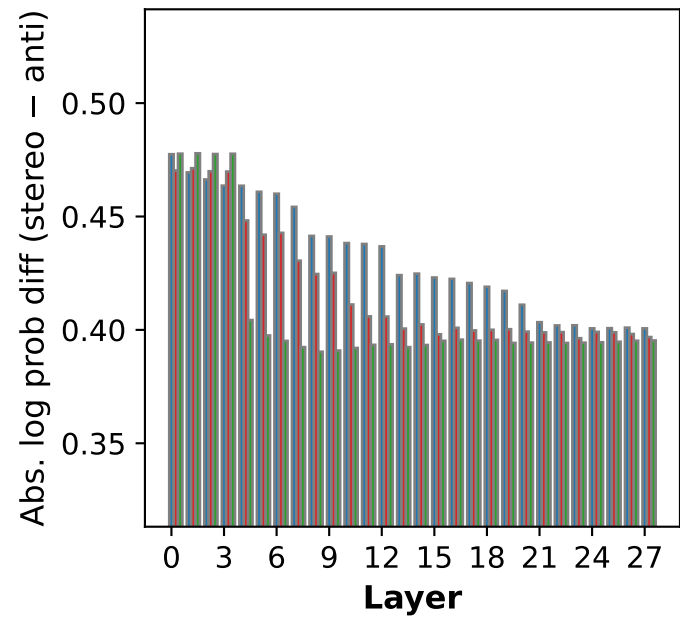
(d) Gender bias effect of different words (Qwen2.5-1.5B)
