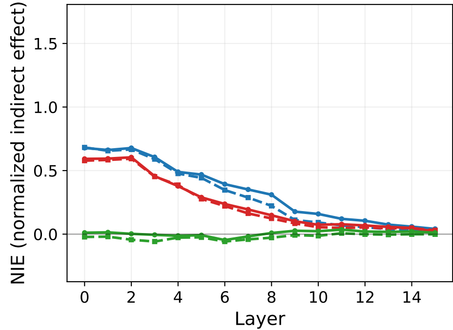
Llama-3.2-1B within-model (solid) vs Llama-3.2-1B-Instruct → Llama-3.2-1B cross-patch (dashed) (j) Gender — Words NIE Llama-3.2-1B within-model (solid) vs Llama-3.2-1B-Instruct → Llama-3.2-1B cross-patch (dashed) (k) Race — Words NIE Llama-3.2-1B within-model (solid) vs Llama-3.2-1B-Instruct → Llama-3.2-1B cross-patch (dashed) (l) Profession — Words NIE
