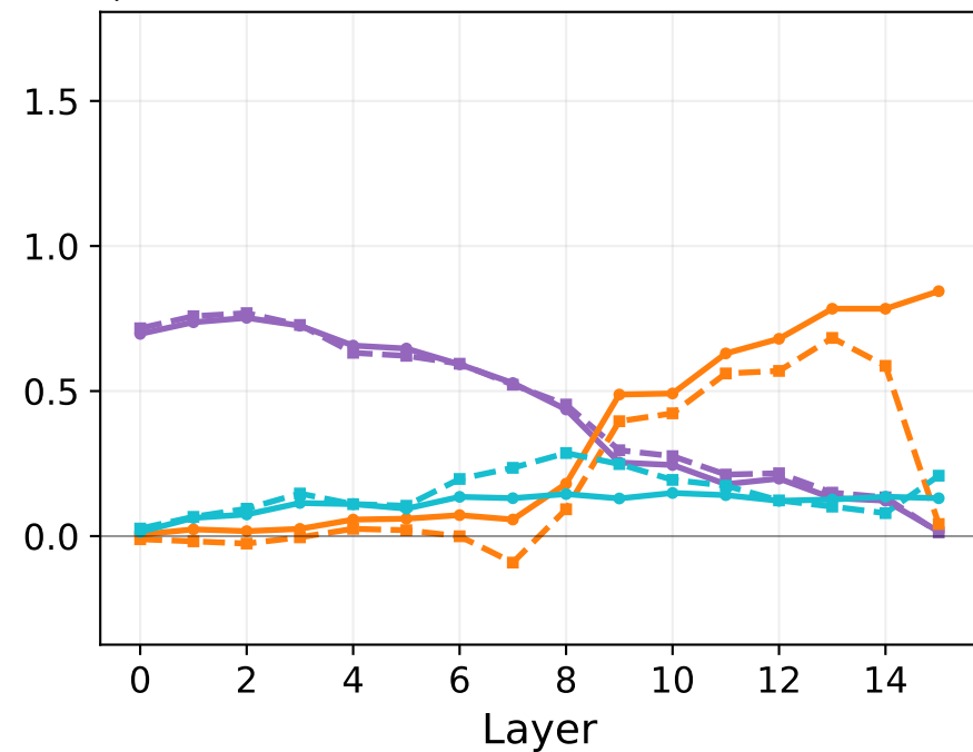
Llama-3.2-1B within-model (solid) vs Llama-3.2-1B-Instruct → Llama-3.2-1B cross-patch (dashed) (g) Gender — States NIE Llama-3.2-1B within-model (solid) vs Llama-3.2-1B-Instruct → Llama-3.2-1B cross-patch (dashed) (h) Race — States NIE Llama-3.2-1B within-model (solid) vs Llama-3.2-1B-Instruct → Llama-3.2-1B cross-patch (dashed) (i) Profession — States NIE
