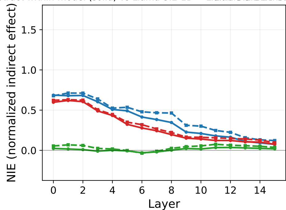
Llama-3.2-1B-Instruct within-model (solid) vs Llama-3.2-1B → Llama-3.2-1B-Instruct cross-patch (dashed) (d) Gender — Words NIE Llama-3.2-1B-Instruct within-model (solid) vs Llama-3.2-1B → Llama-3.2-1B-Instruct cross-patch (dashed) (e) Race — Words NIE Llama-3.2-1B-Instruct within-model (solid) vs Llama-3.2-1B → Llama-3.2-1B-Instruct cross-patch (dashed) (f) Profession — Words NIE
