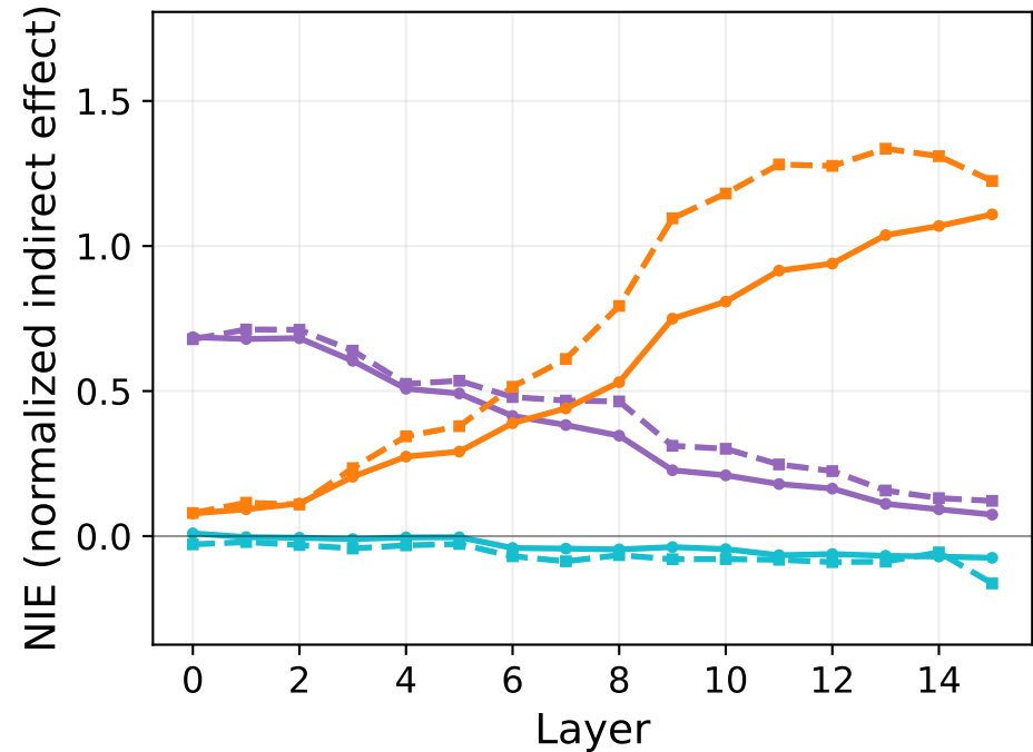
Llama-3.2-1B within-model (solid) vs Llama-3.2-1B-Instruct → Llama-3.2-1B cross-patch (dashed) (g) Gender — States NIE Llama-3.2-1B within-model (solid) vs Llama-3.2-1B-Instruct → Llama-3.2-1B cross-patch (dashed) (h) Race — States NIE Llama-3.2-1B within-model (solid) vs Llama-3.2-1B-Instruct → Llama-3.2-1B cross-patch (dashed) (i) Profession — States NIE
