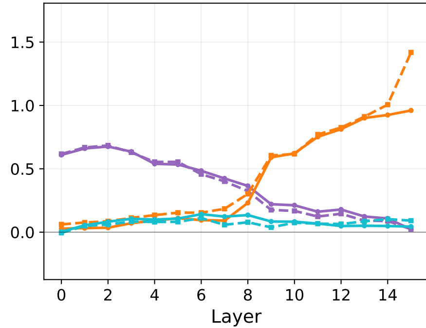
Llama-3.2-1B within-model (solid) vs Llama-3.2-1B-Instruct → Llama-3.2-1B cross-patch (dashed) (j) Gender — Words NIE Llama-3.2-1B within-model (solid) vs Llama-3.2-1B-Instruct → Llama-3.2-1B cross-patch (dashed) (k) Race — Words NIE Llama-3.2-1B within-model (solid) vs Llama-3.2-1B-Instruct → Llama-3.2-1B cross-patch (dashed) (l) Profession — Words NIE
