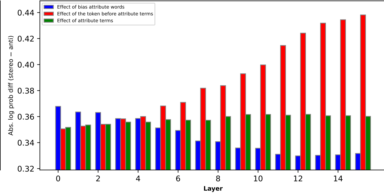
step1400
