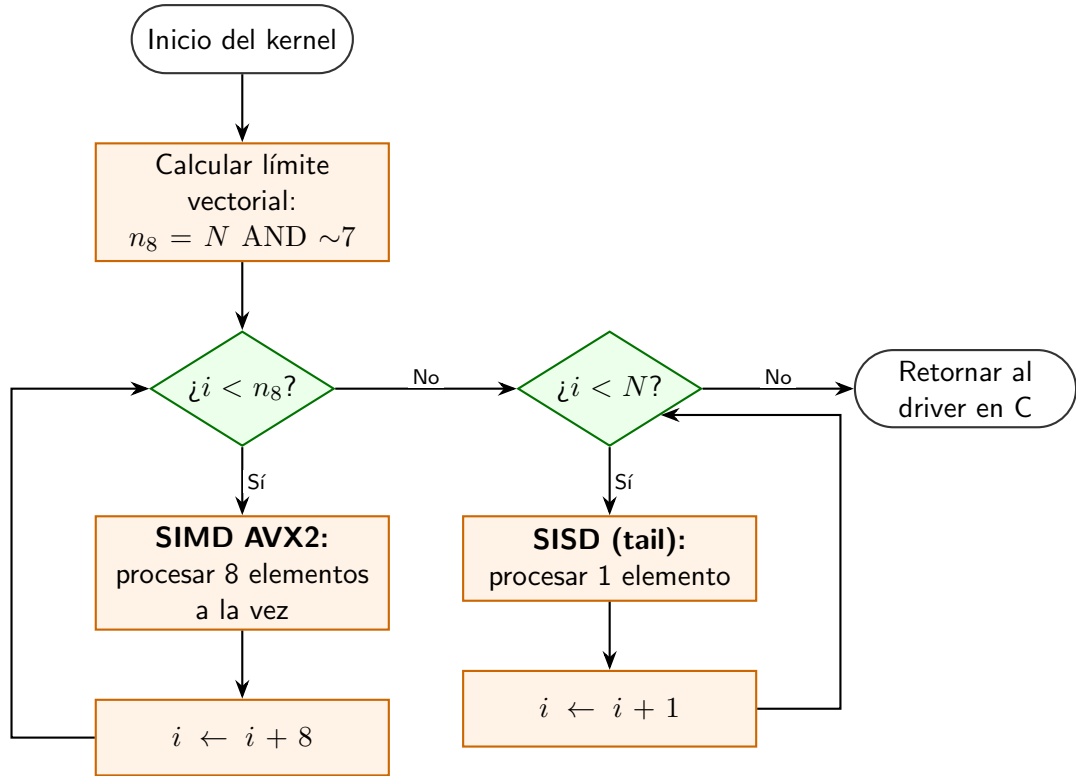
Figura 3: Diagrama de flujo mostrando la transición al bucle remanente ( tail loop ).
