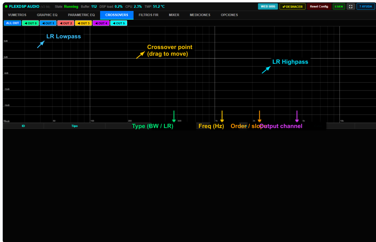
Active crossovers with frequency response graph / Crossovers activos con gráfico de respuesta en frecuencia
