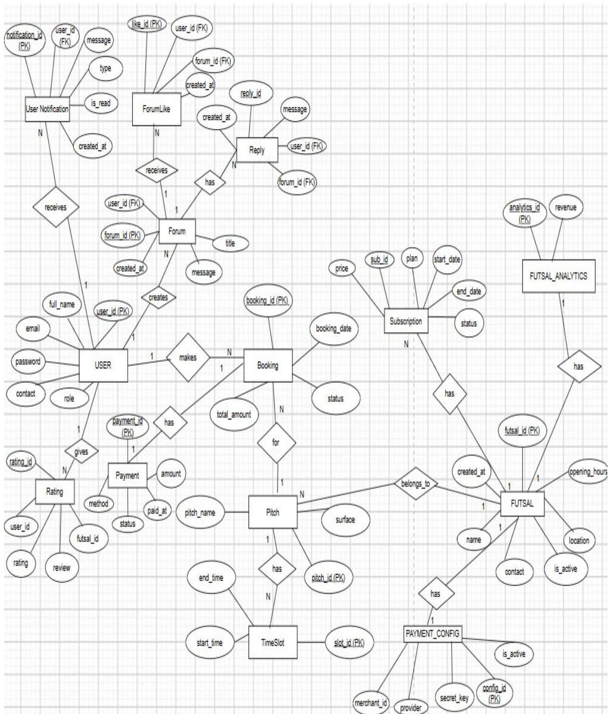
Figure 3.4 : ER Diagram
