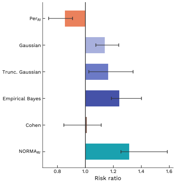
eICU-CRD
