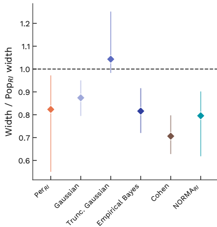
Interval width
