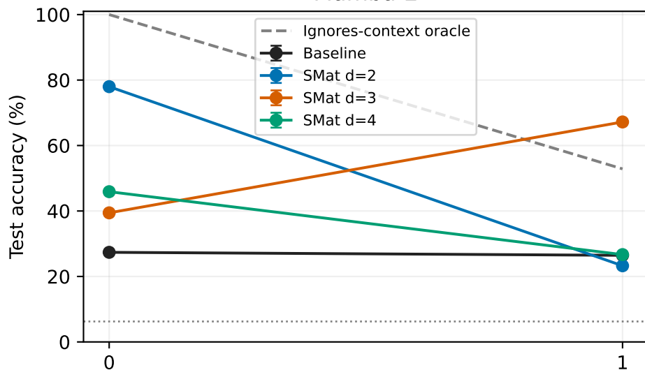
Mamba-2
