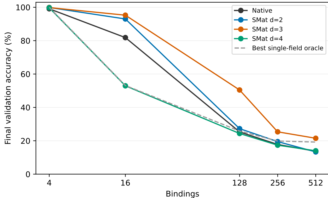
mamba2
