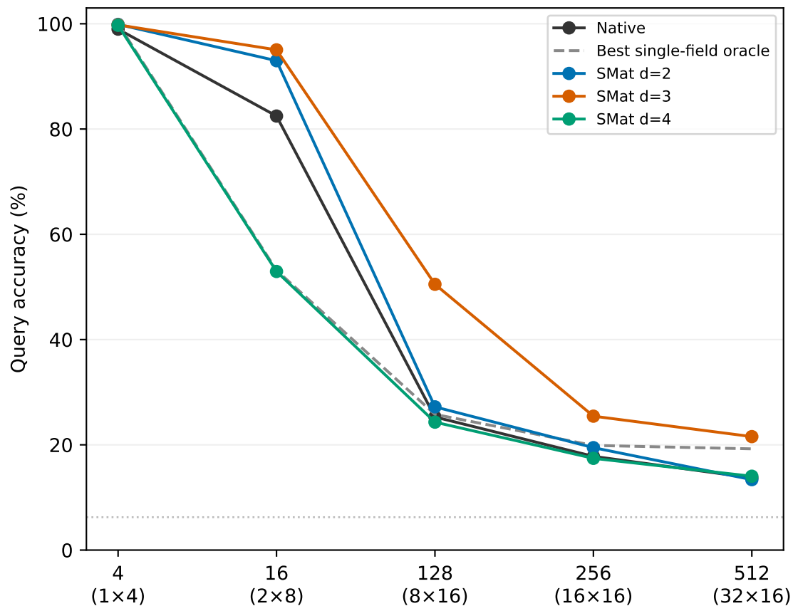
Mamba-2
