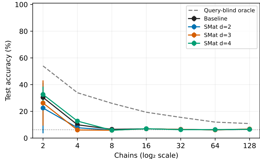
Mamba-2
