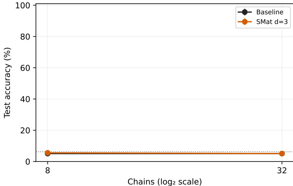
Mamba-2
