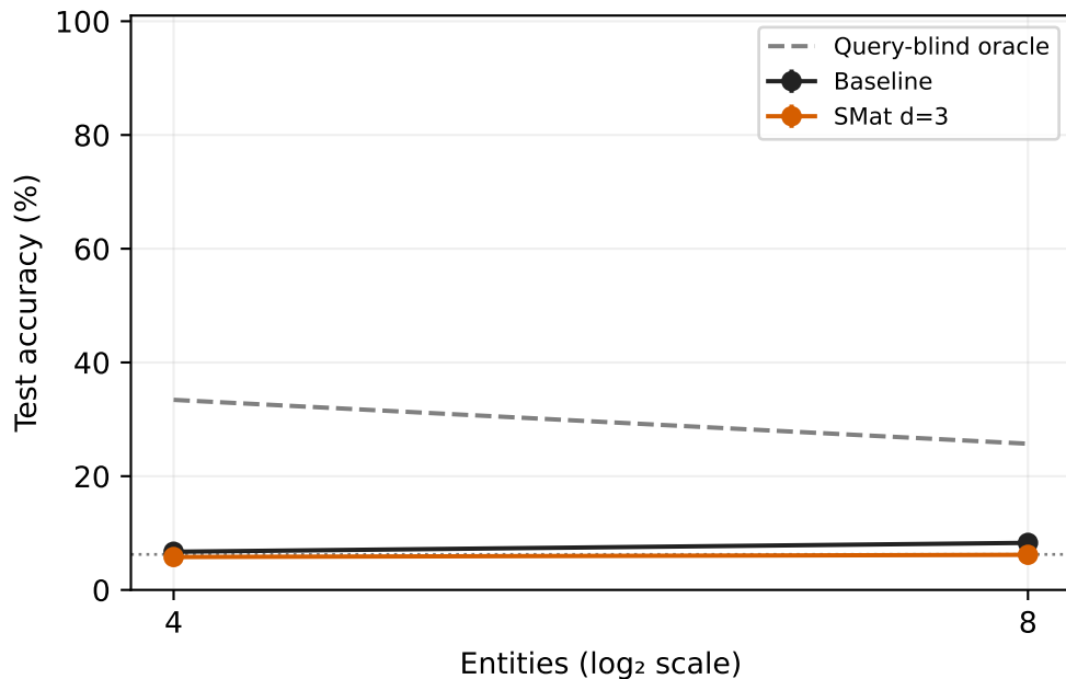
Mamba-2
