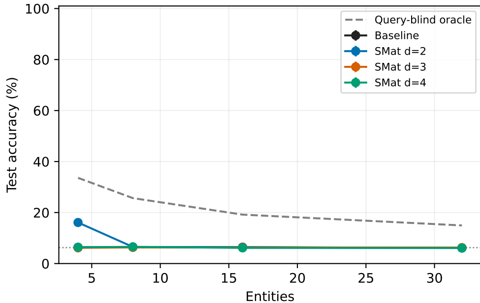
mamba2
