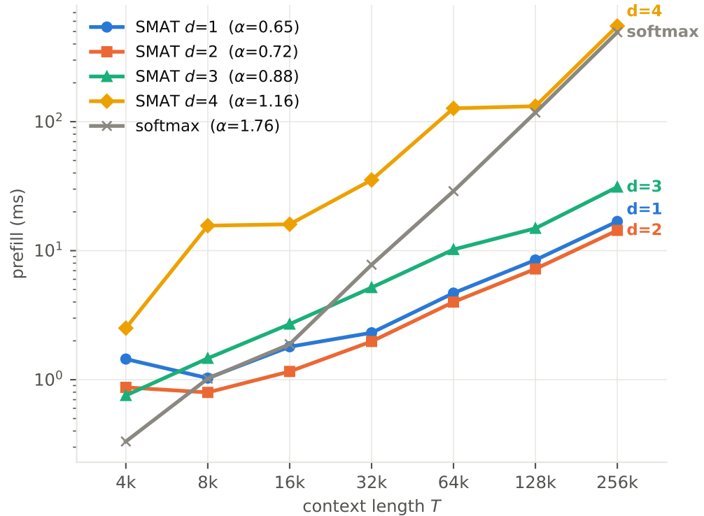
Prefill cost, one layer
