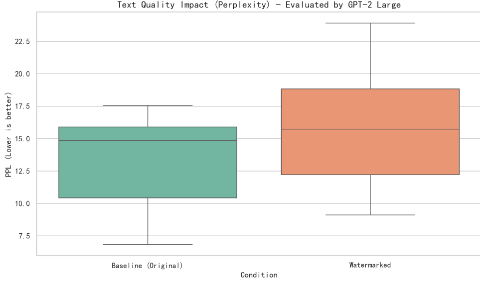
Figure 1: 水印植入对文本自然度 (PPL) 的影响。箱线图展示了 Baseline 与 Watermarked 文本的困惑度分布差异，水印导致 PPL 均值从 11.45 上升至 15.32 ( \uparrow 33.8\% )，表明 Logit 偏置对生成质量存在不可忽略的负面影响。
