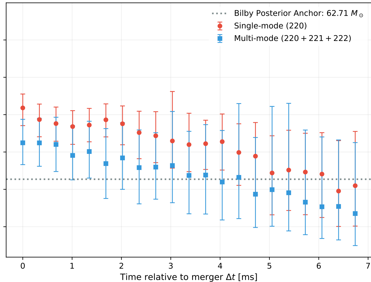
(b) Real Event GW250114 Parameter Evolution
