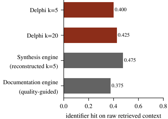
Raw retrieval
