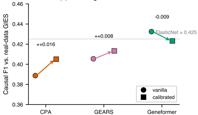
(b) F1 change after calibration
