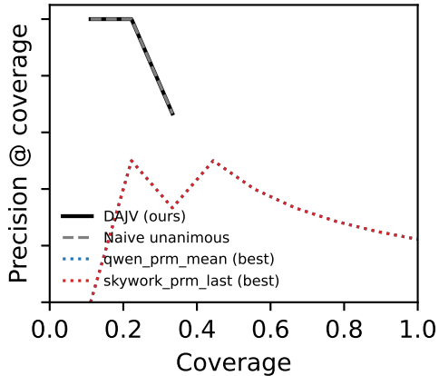
Bench: aime
