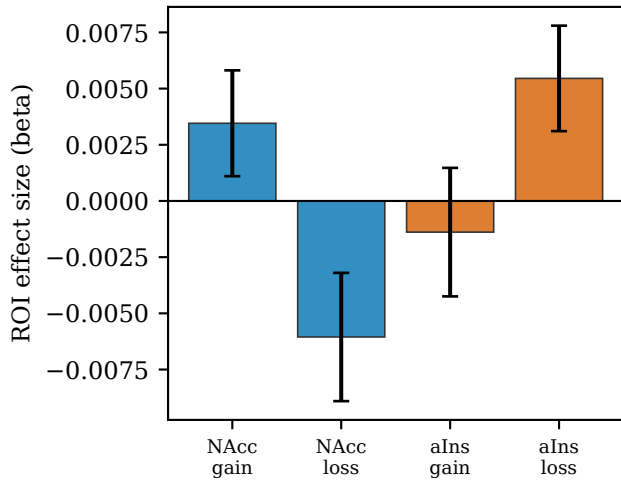
real NARPS fMRI (n=40)
