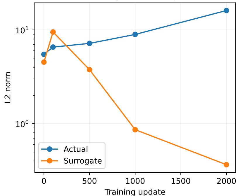
Parameter-gradient magnitude
