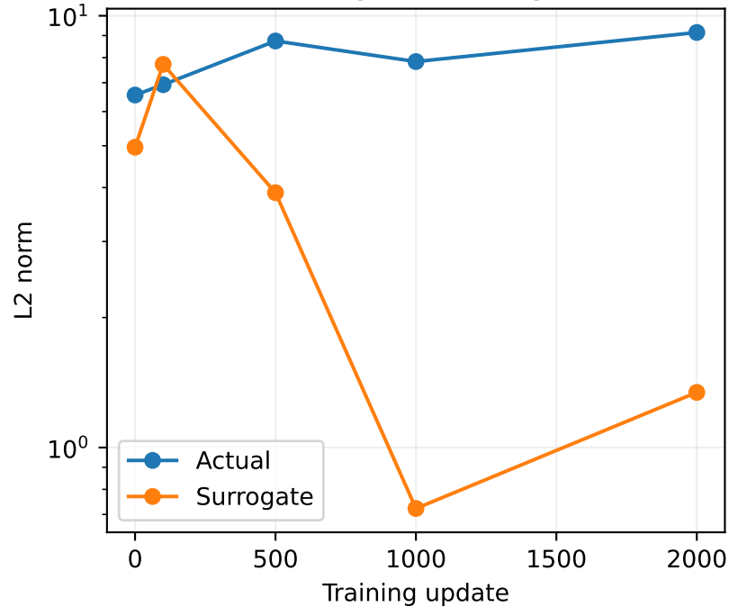
Parameter-gradient magnitude
