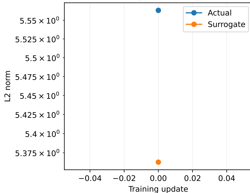
Parameter-gradient magnitude
