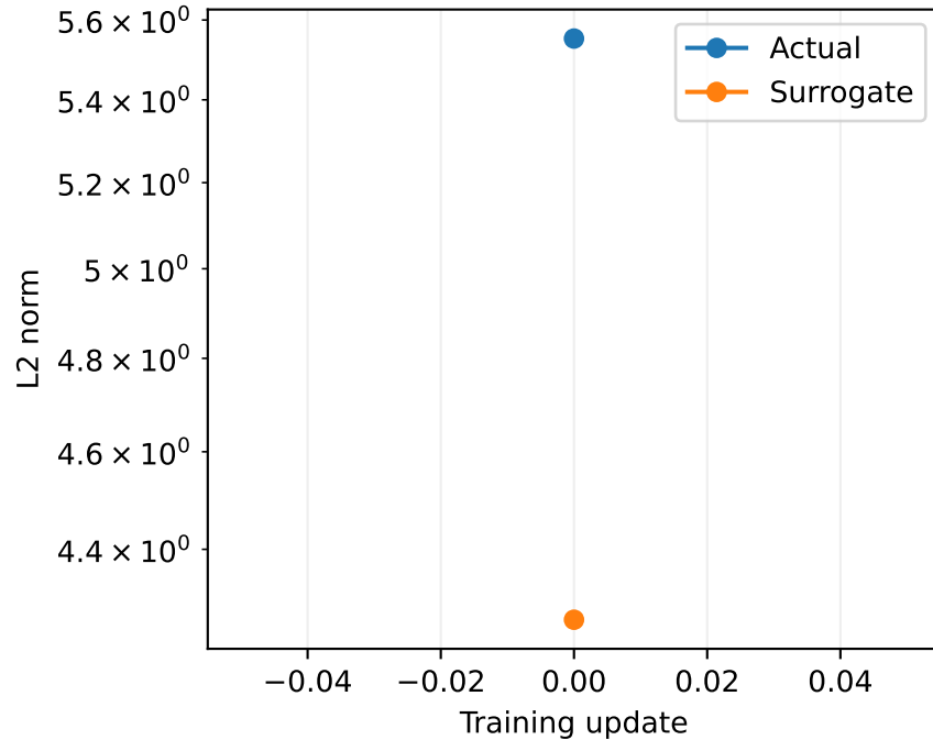
Parameter-gradient magnitude
