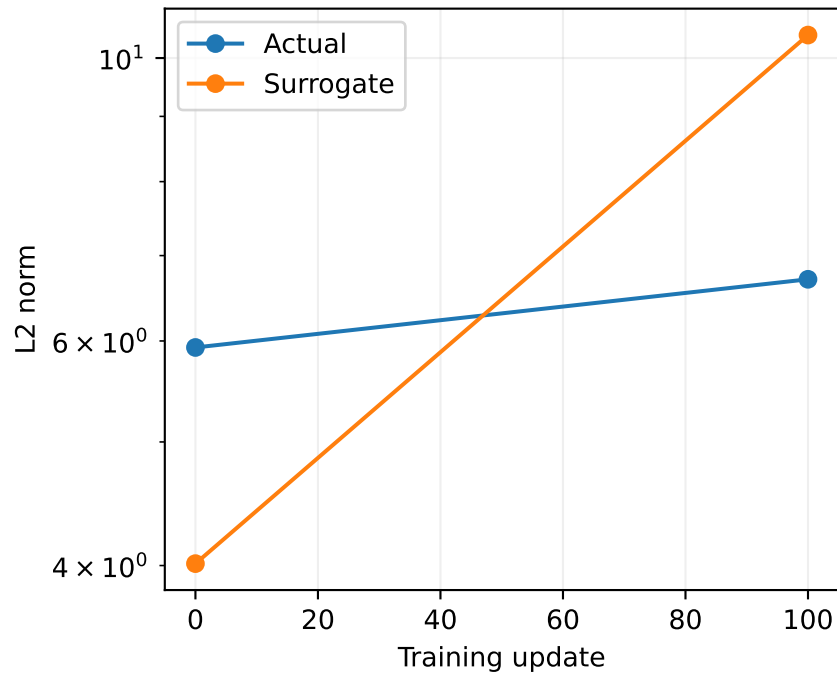
Parameter-gradient magnitude
