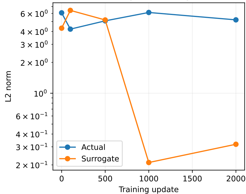
Parameter-gradient magnitude
