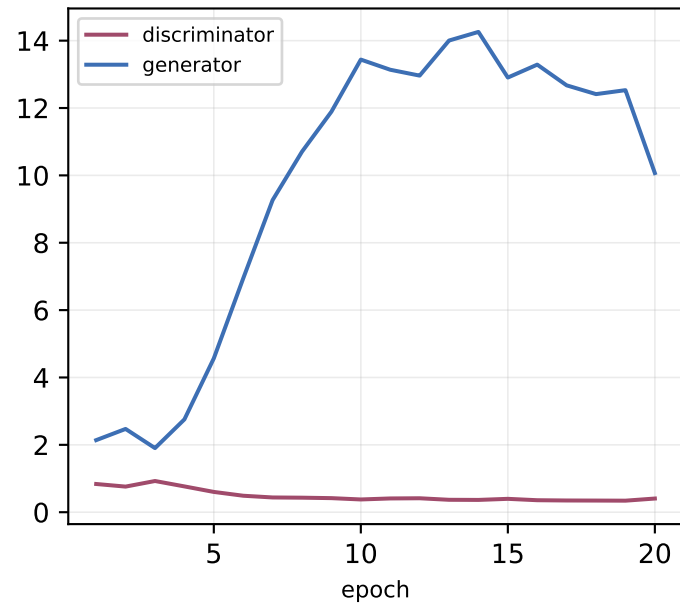
GAN
