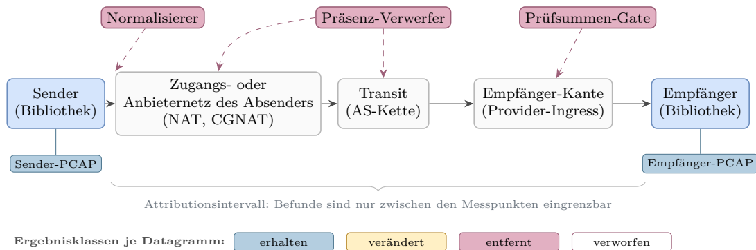
Abbildung 4.3: Kantenmodell eines Messpfads mit den erwarteten Mechanismenklassen
