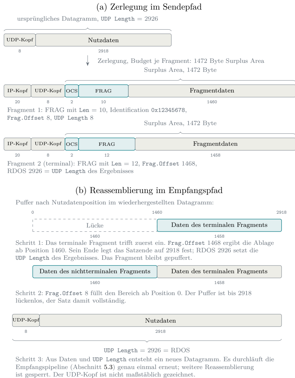
Abbildung 5.4: Zerlegung und Reassemblierung eines Datagramms mit 2918 Nutzdatenbytes
