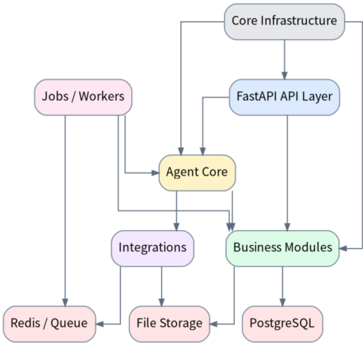
图：12.2 后端模块化单体架构
