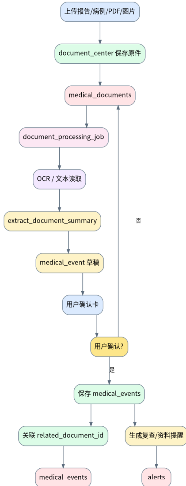
图：12.7 文档处理链路
