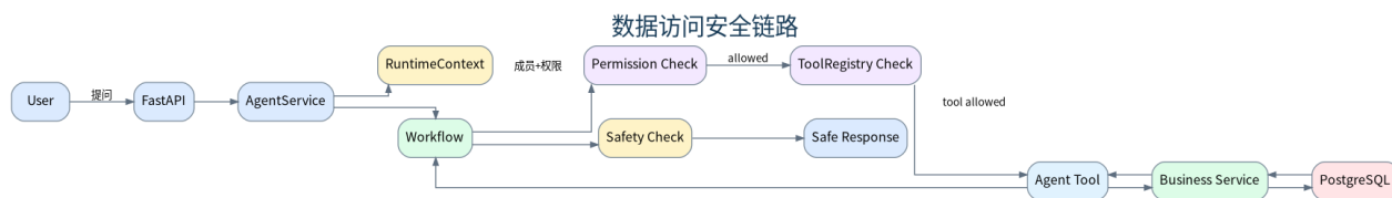
图：12.5 数据访问安全链路
