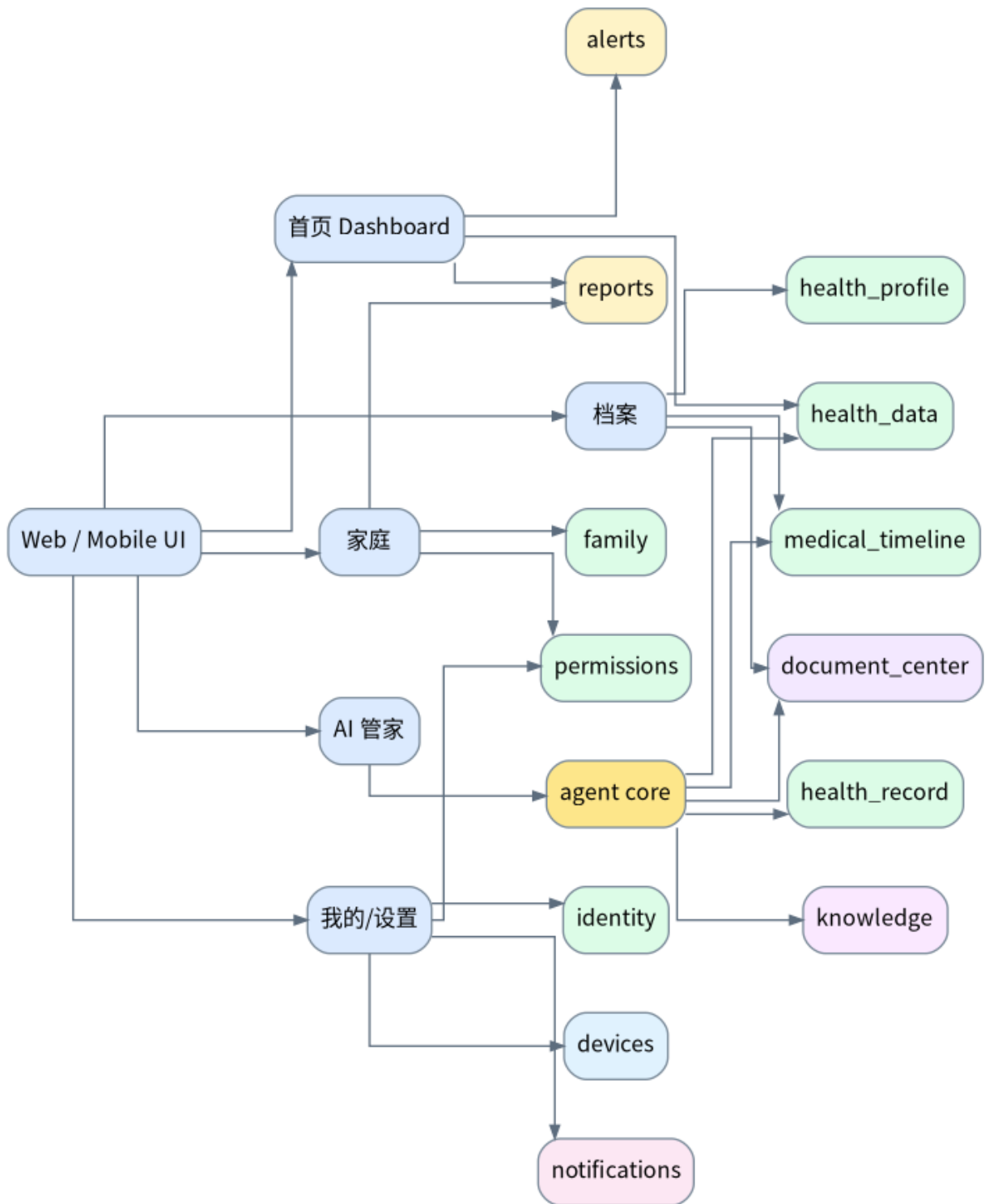
图：12.9 前端页面与后端模块映射
