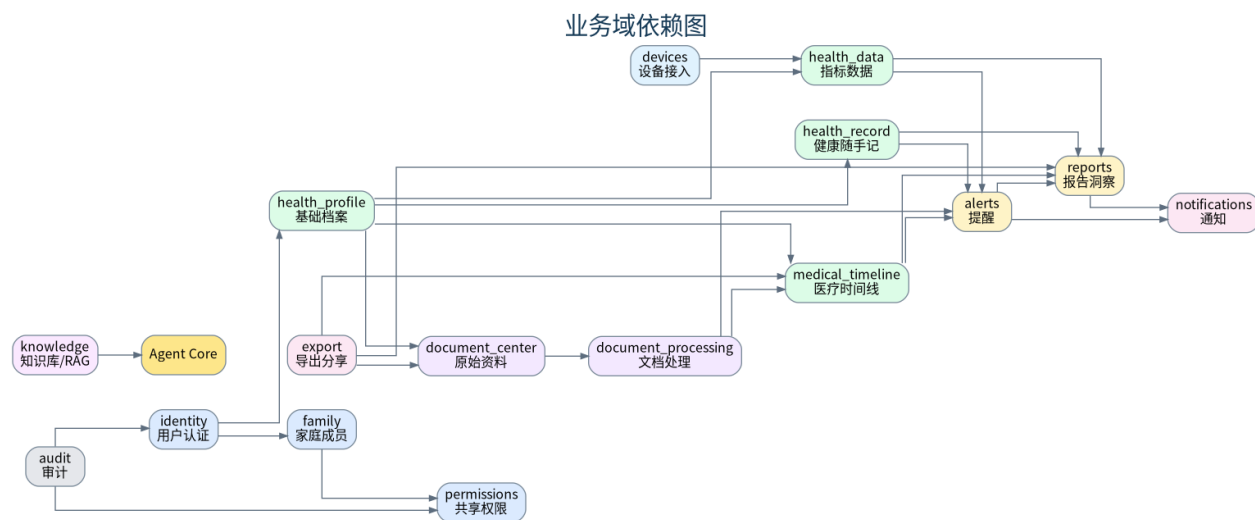
图：12.3 业务域依赖图
