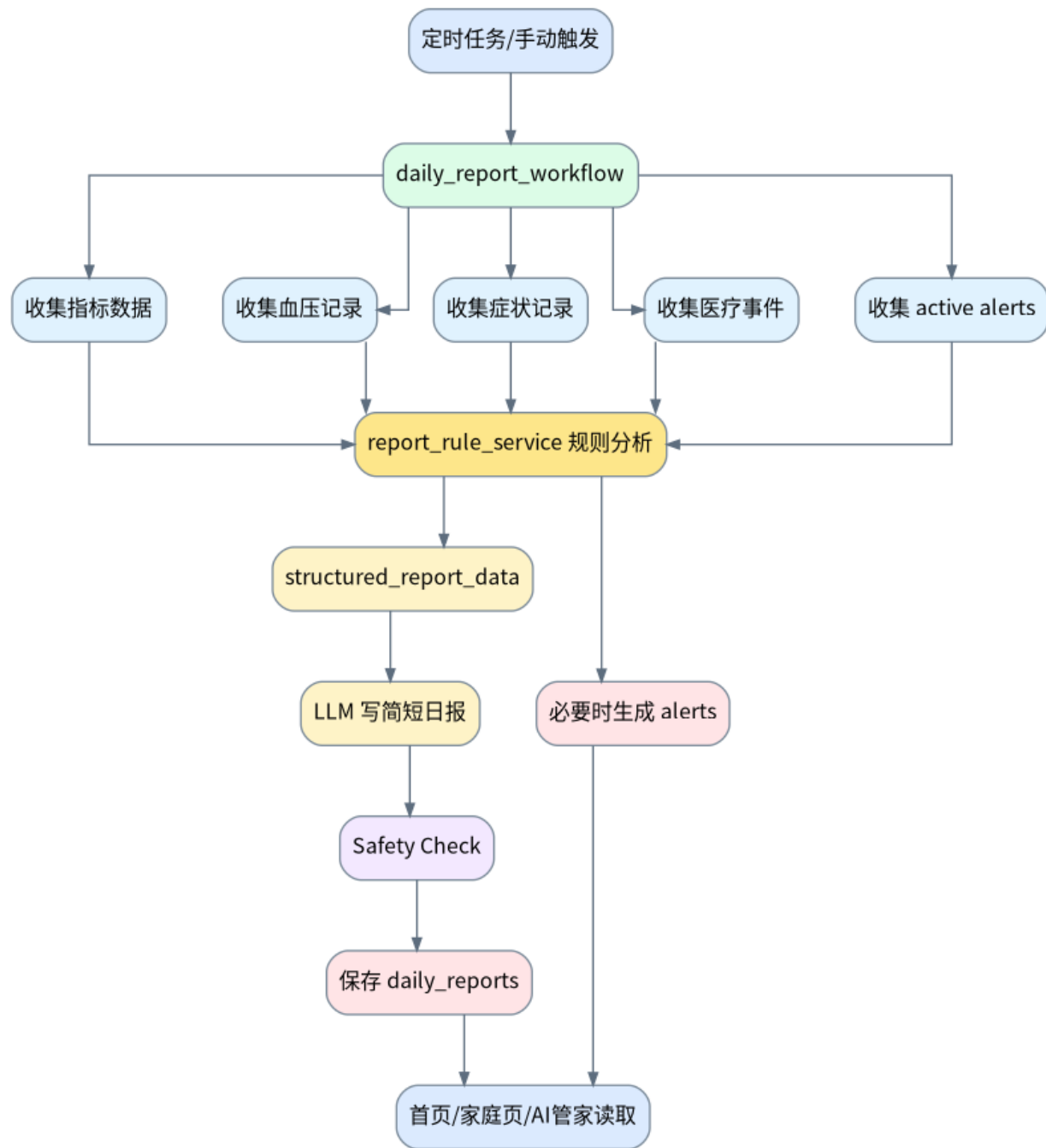
图：12.8 日报生成链路
