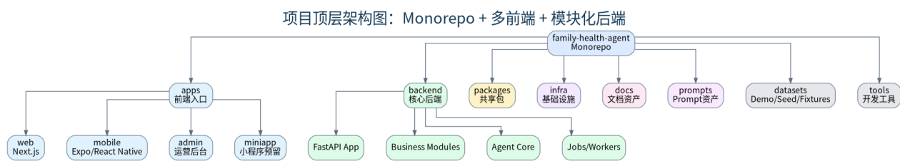
图：12.1 项目顶层架构图
