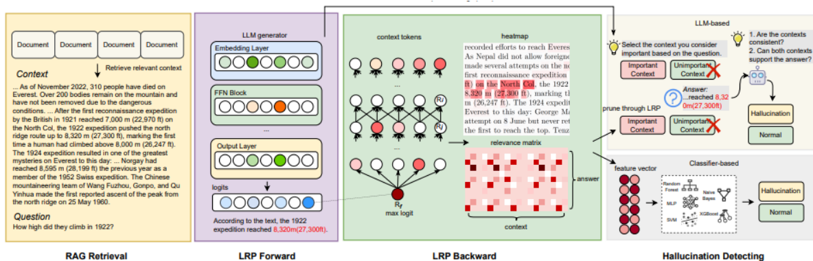
Slika 11: Arhitektura LRP4RAG metode za otkrivanje halucinacija [47]
