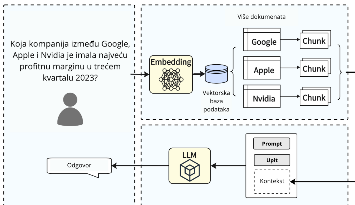
Slika 12: Višeskočno zaključivanje - primjer [49]
