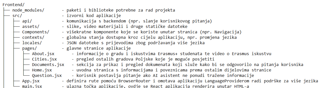
Slika 23: Struktura frontend dijela
