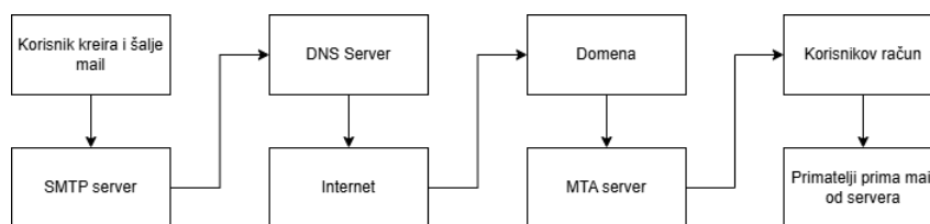
Slika 17: Proces dostavljanja emaila [60]
