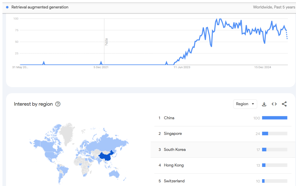
Slika 6: Popularnost RAG-a [30]
