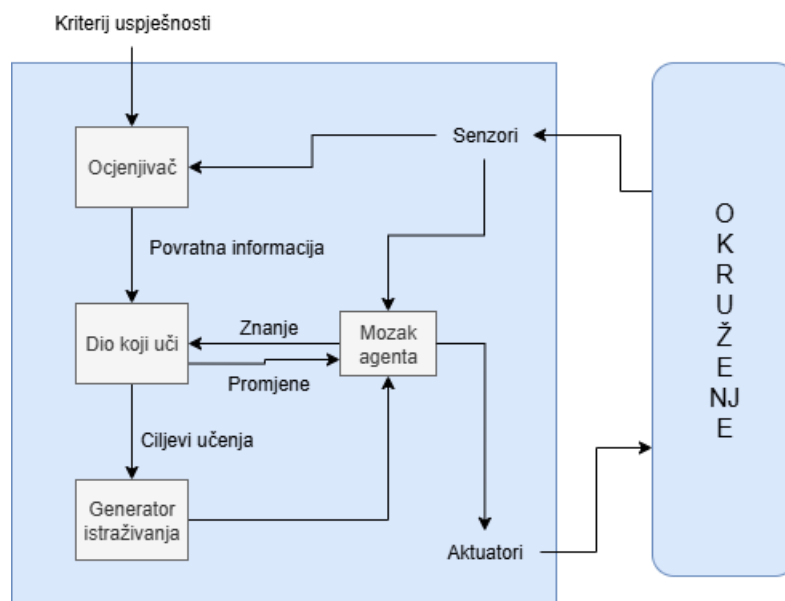
Slika 1: Opći učeći agent – objašnjenje; [9, str. 74]
