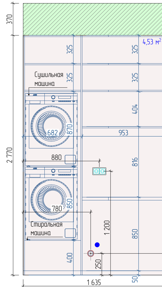
Б-02 Развертка стены 1:25
