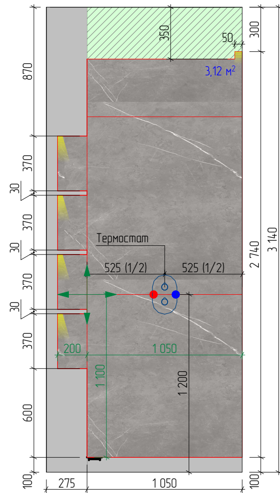
Г-04 Развертка стены 1:25
