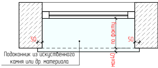
Схема монтажа подоконника
