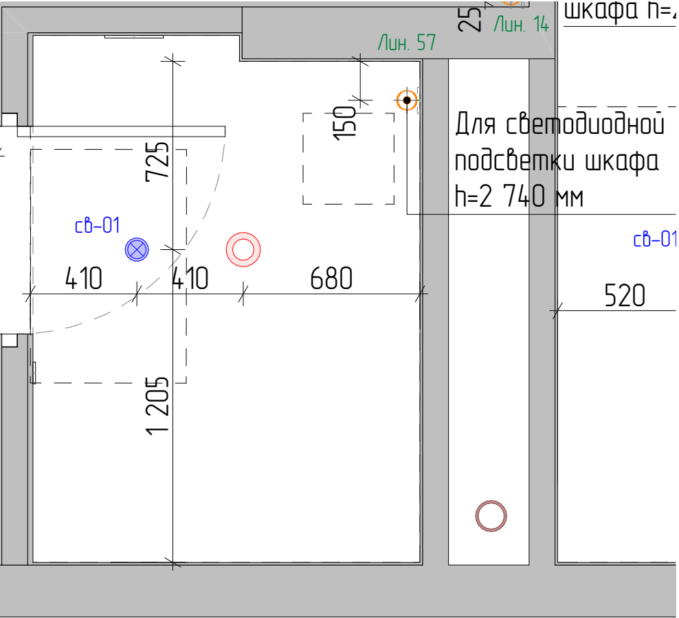
План размещения освещения и выключателей:
