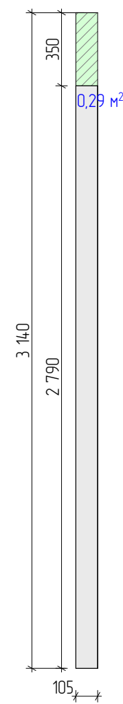
Е-05 Развертка стены 1:25
