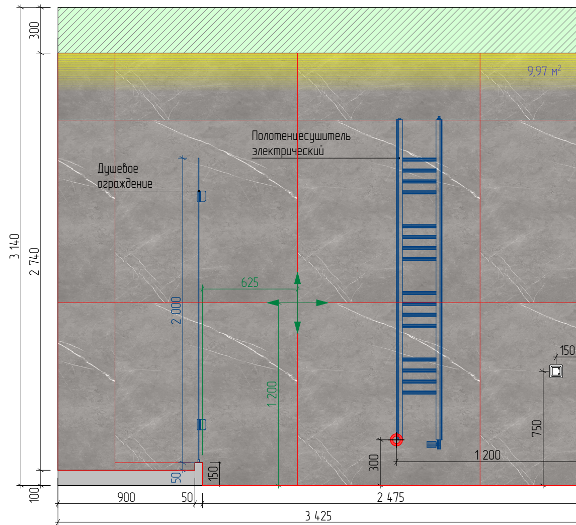
Г-05 Развертка стены 1:25
