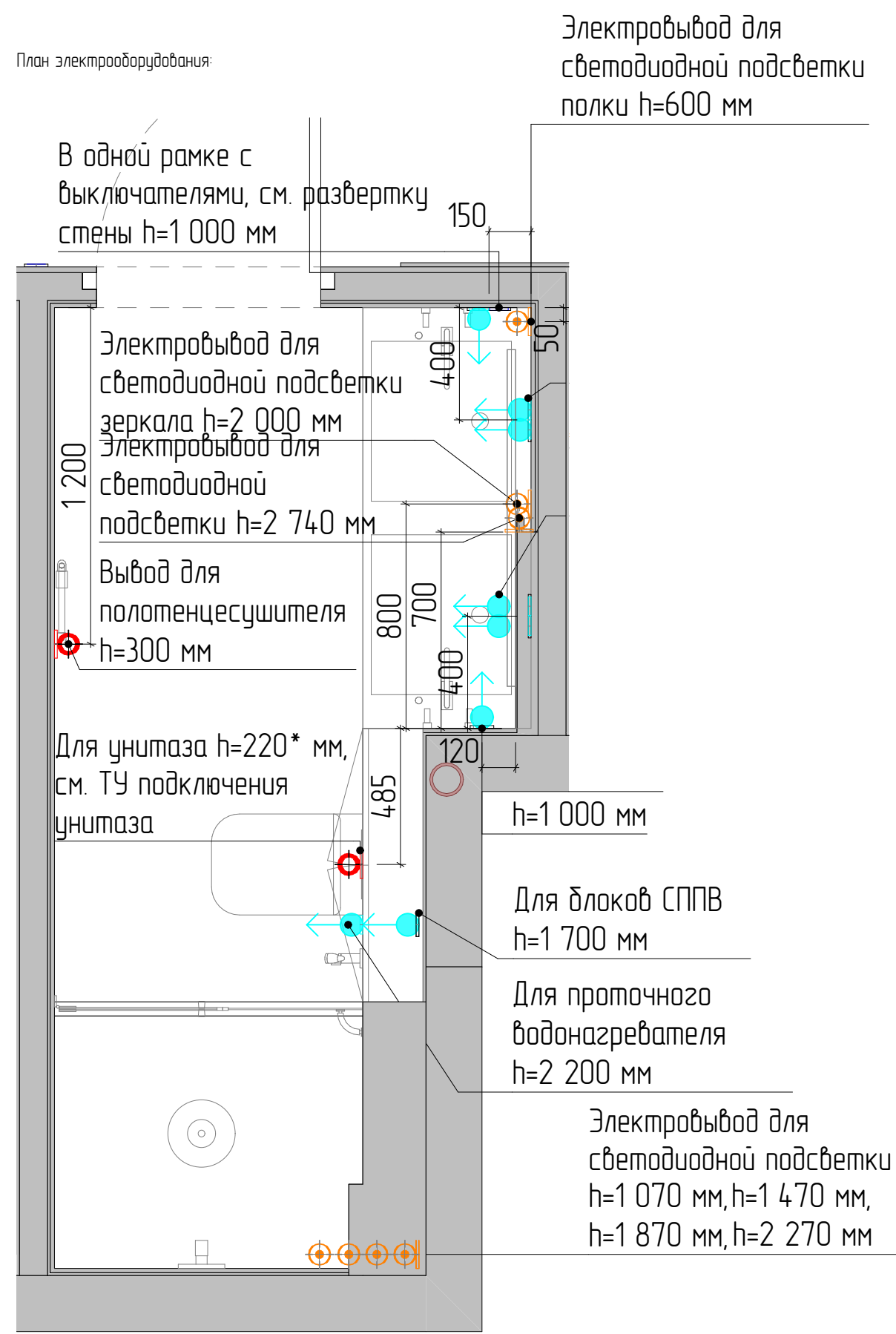
План размещения освещения и выключателей:
