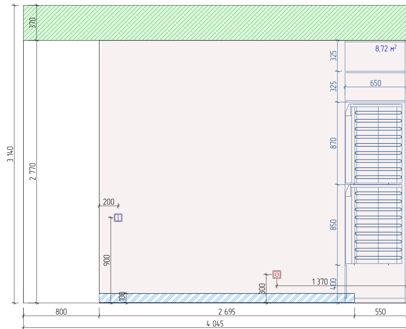
Б-01 Развертка стены 1:25
