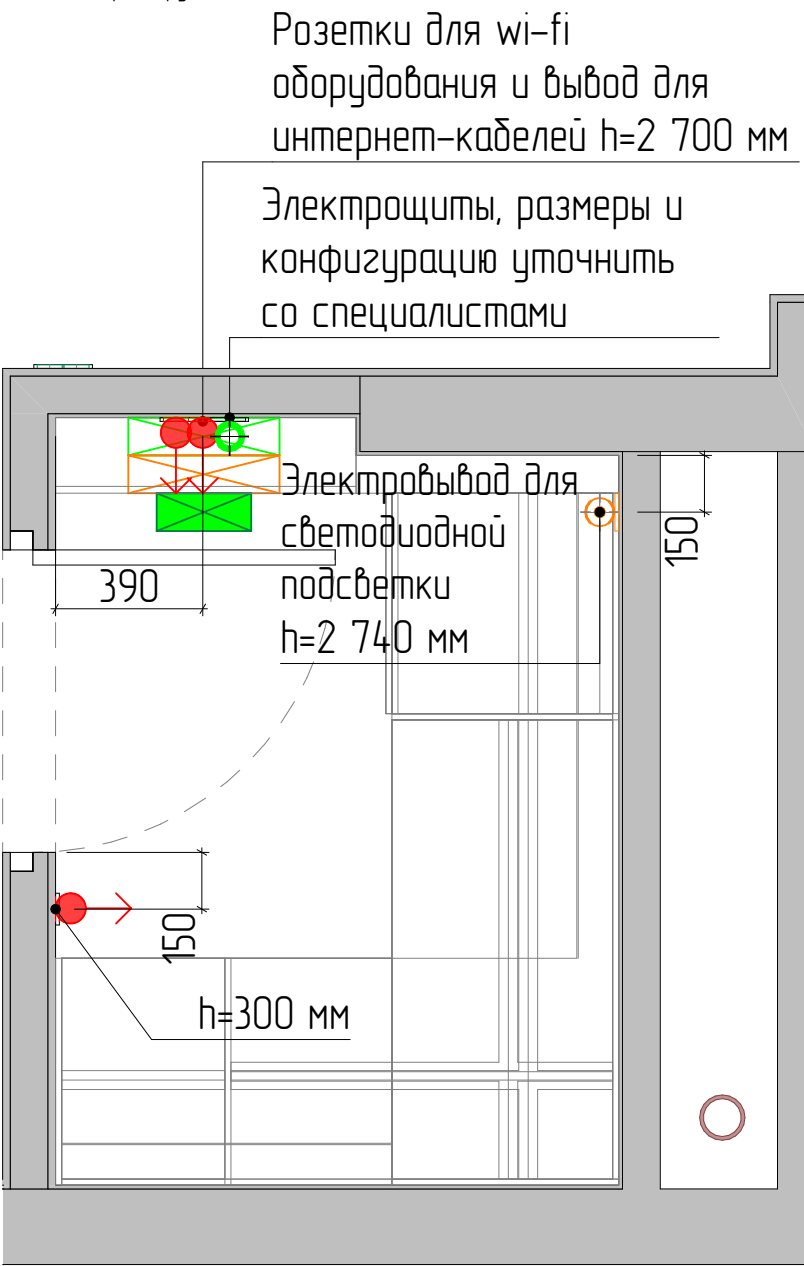
План электрооборудования:
