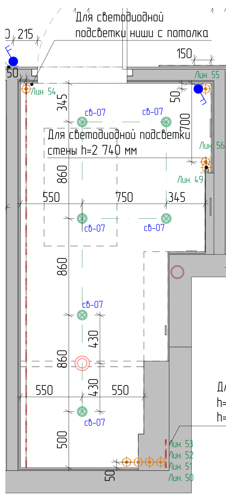
План размещения освещения и выключателей:
