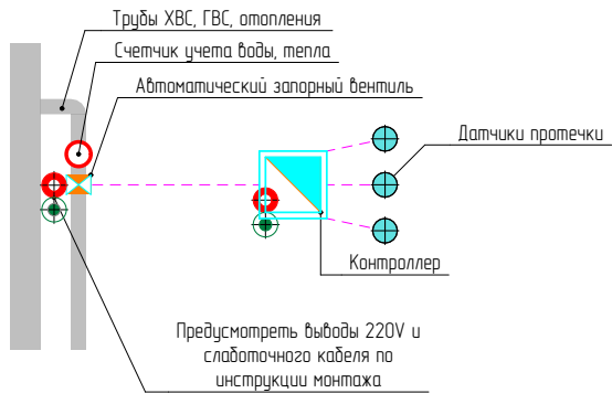
Схема подключения системы датчиков протечки воды.
