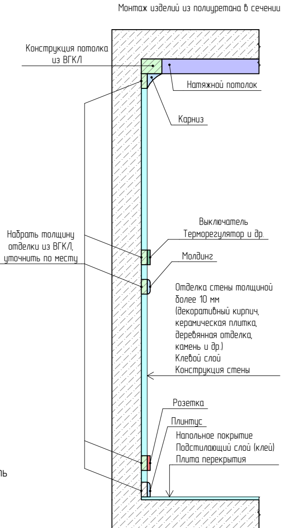
Узел монтажа натяжного потолка к стене с отделкой керамической плиткой.
