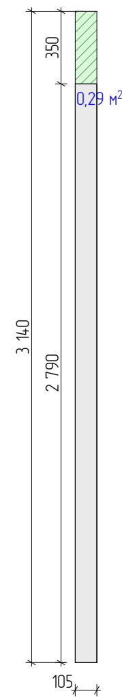
Е-05 Развертка стены 1:25
