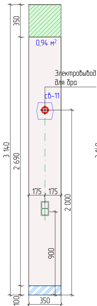
И-07 Развертка стены 1:25
