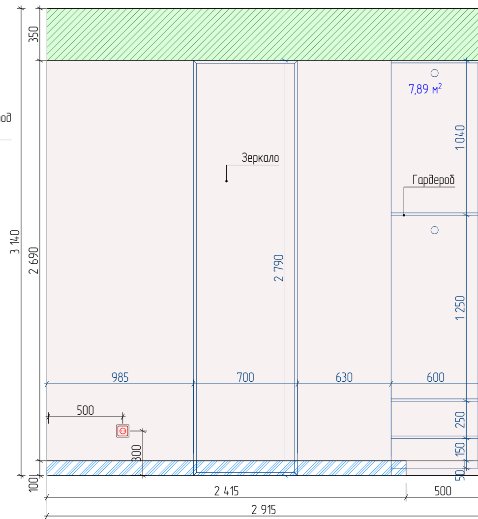
И-08 Развертка стены 1:25
