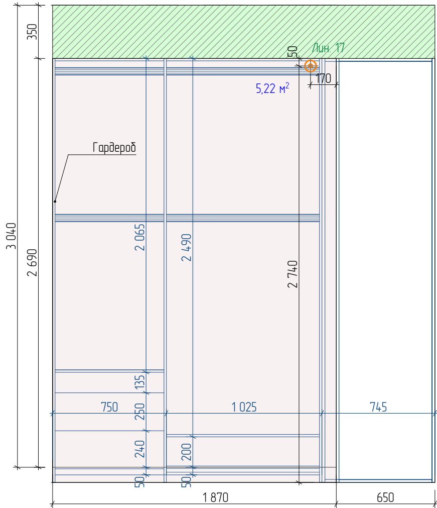
И-02 Развертка стены 1:25
