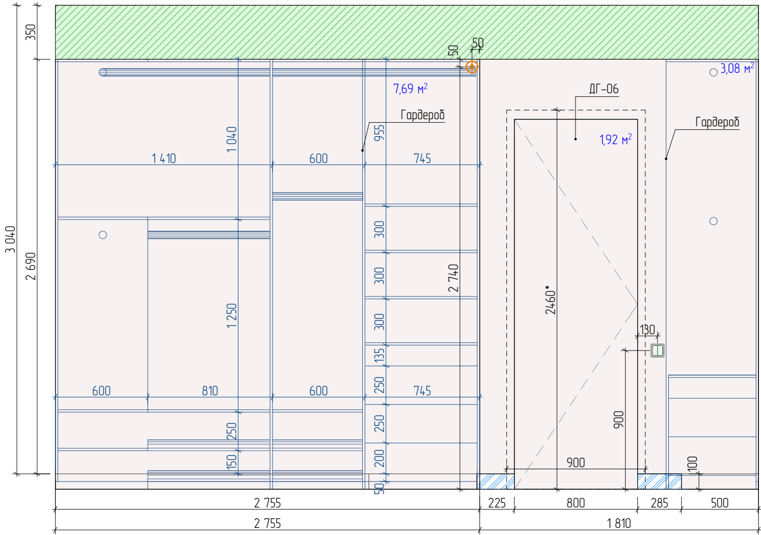
И-01 Развертка стены 1:25
