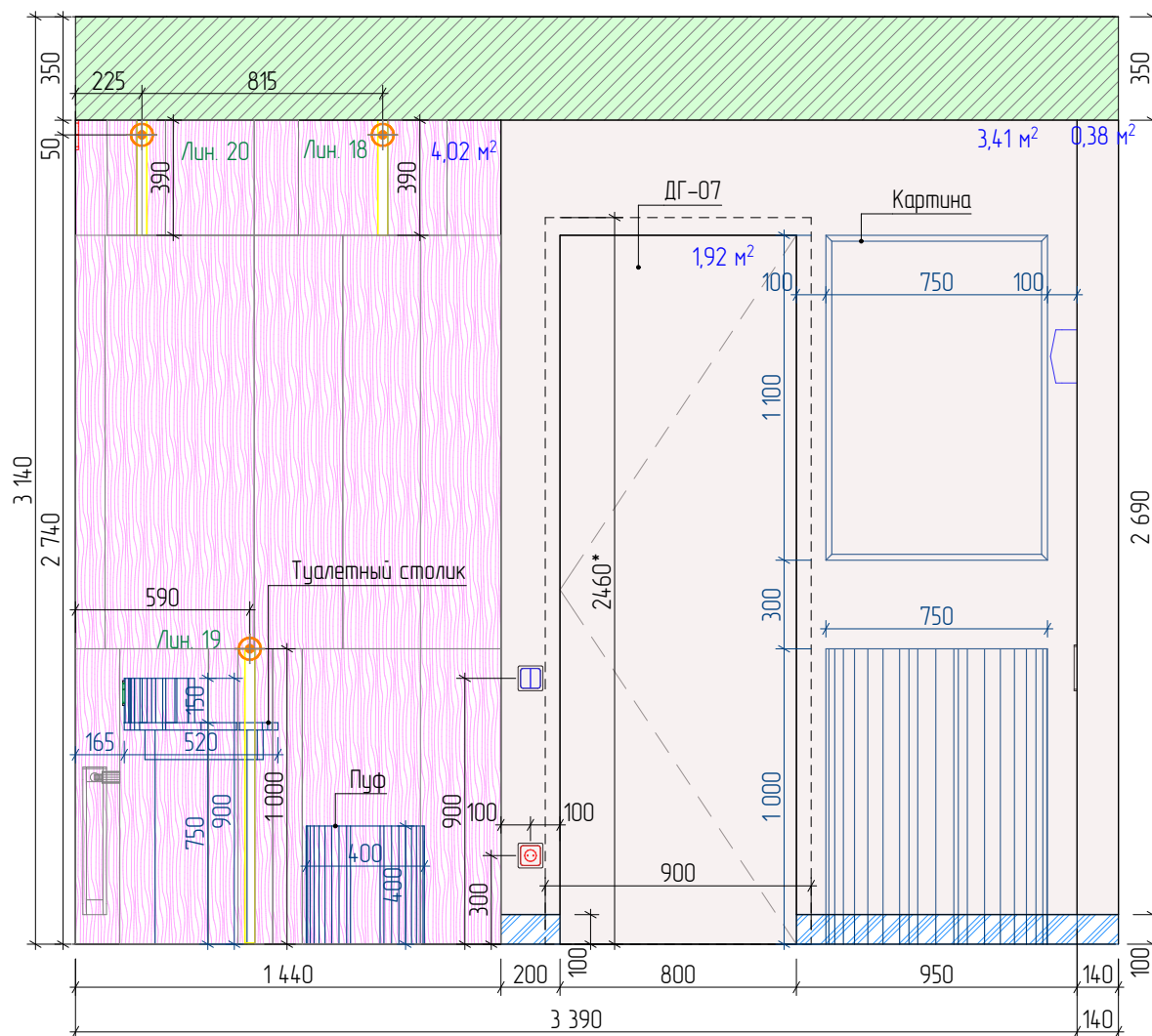
И-10 Развертка стены 1:25
