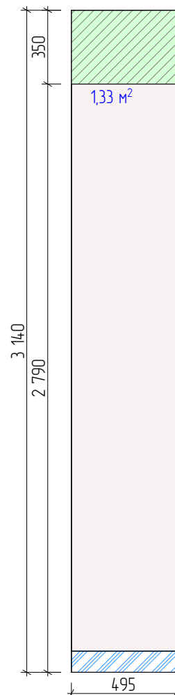
И-10 Развертка стены 1:25
