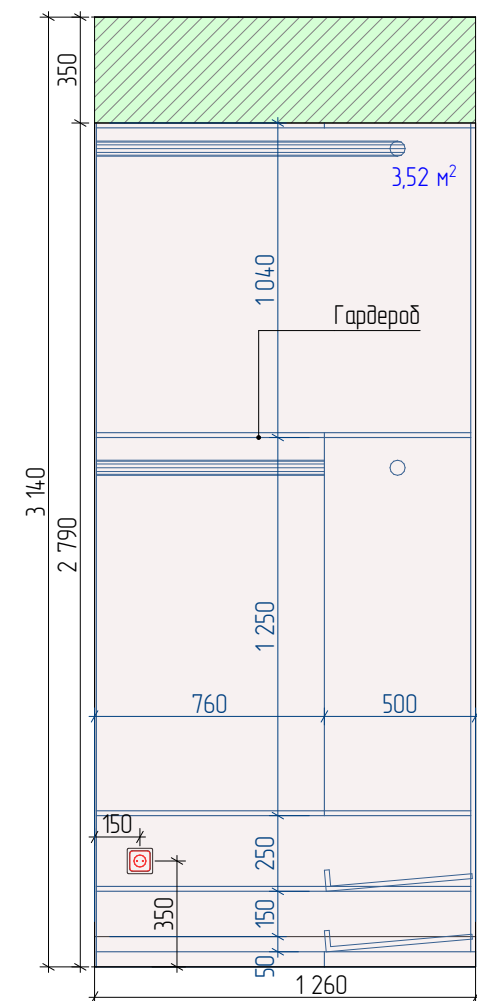
И-09 Развертка стены 1:25
