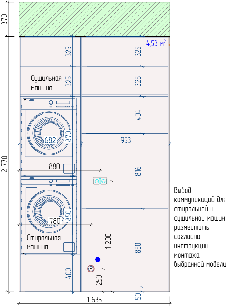
Б-02 Развертка стены 1:25
