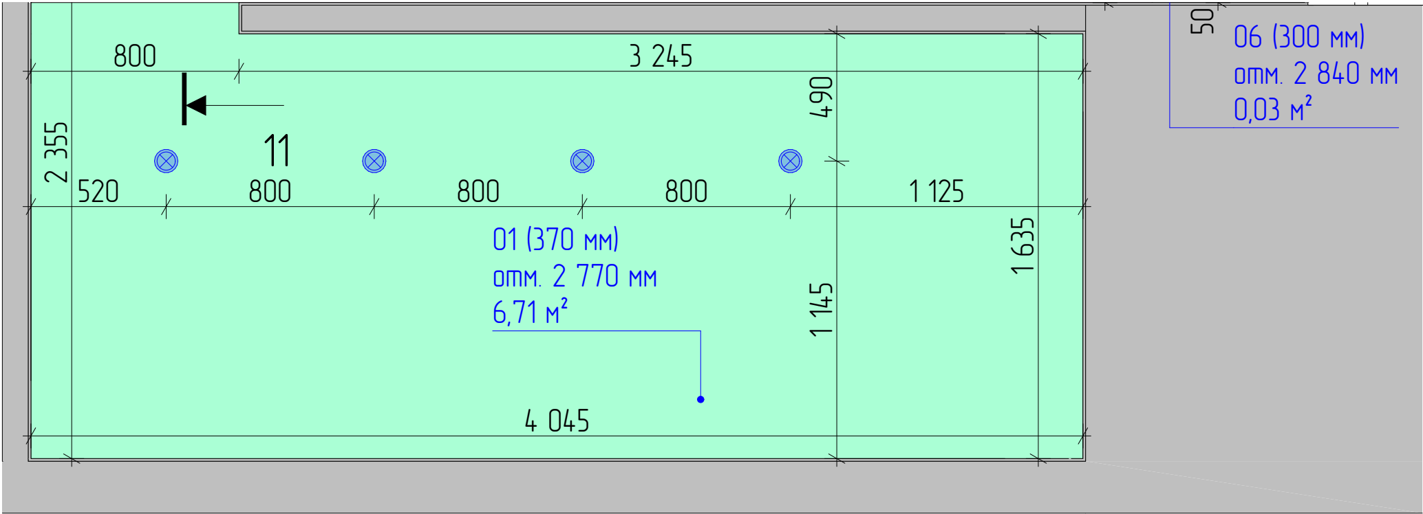
План отделки потолка:
