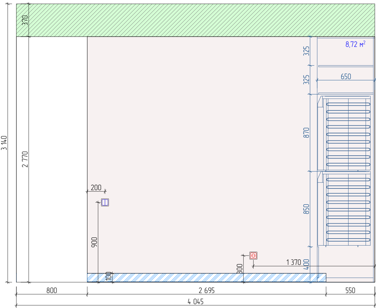
Б-01 Развертка стены 1:25
