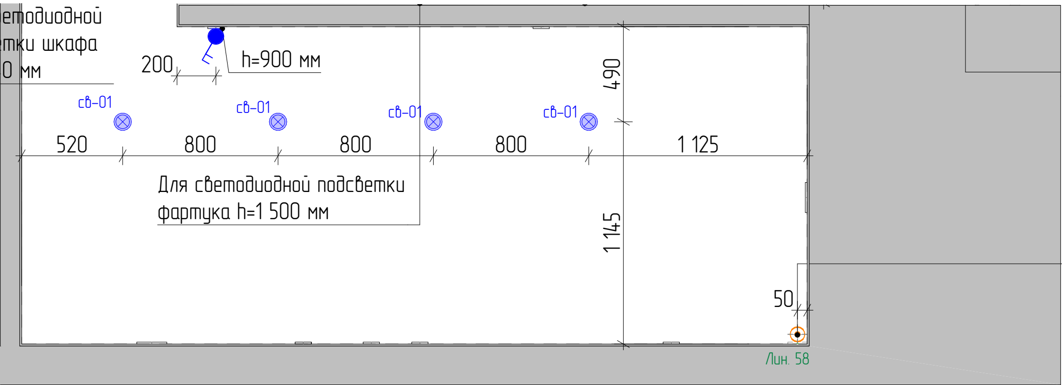
План размещения освещения и выключателей:
