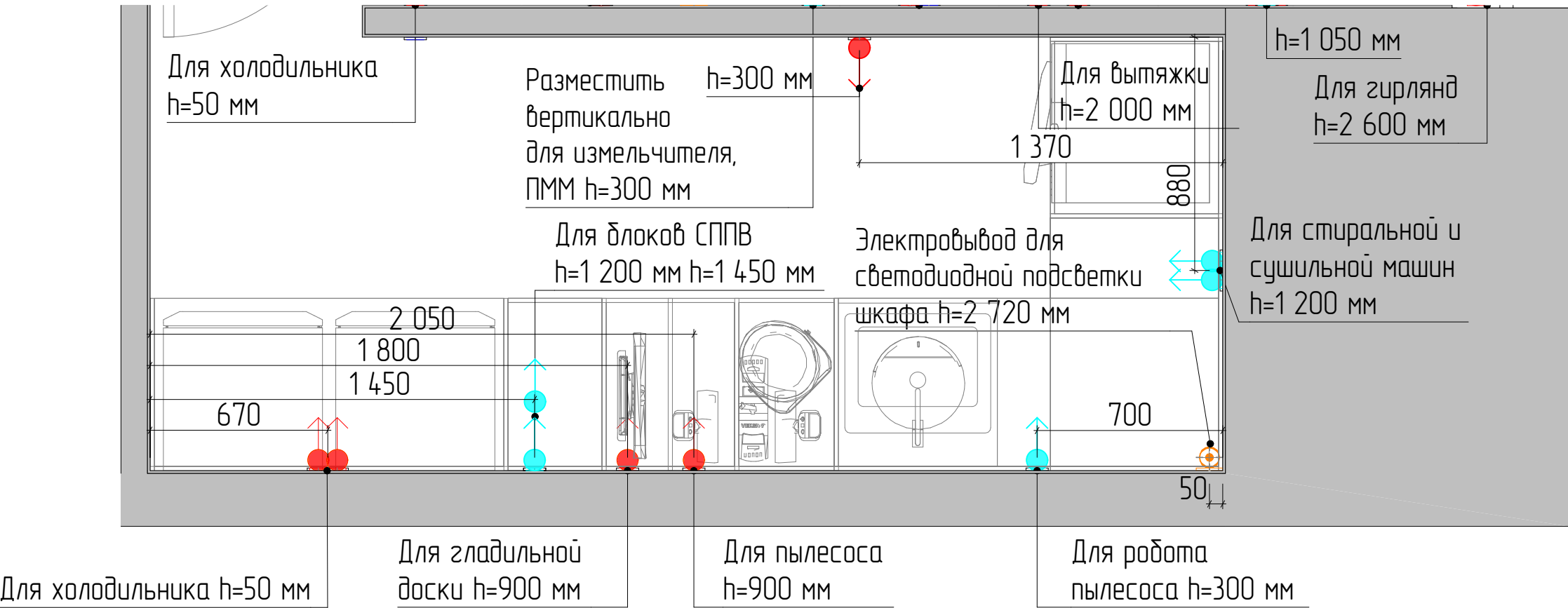
План электрооборудования:
