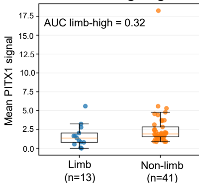
D. PITX1 average signal
