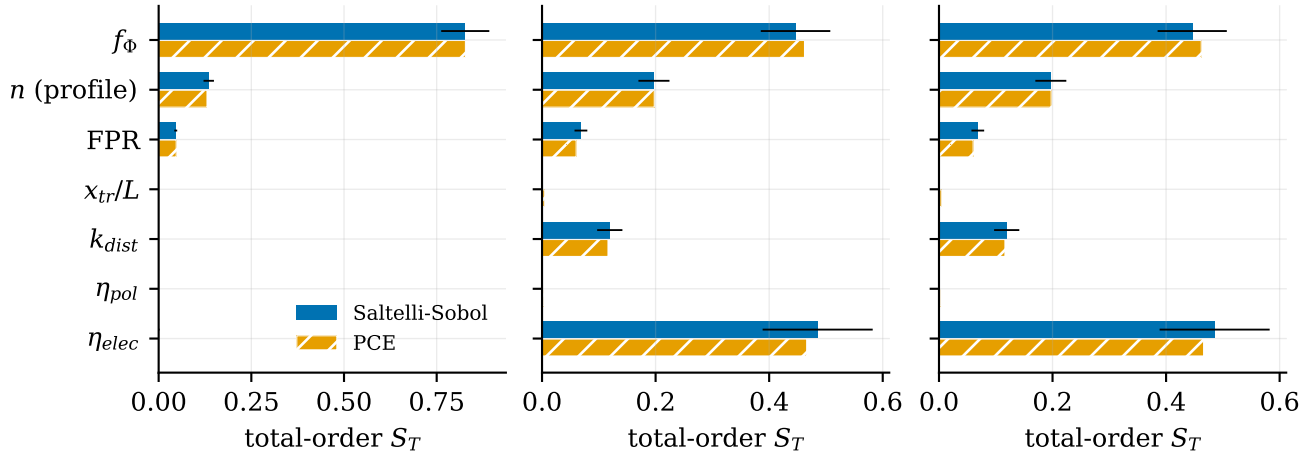
PSC aero (subsystem)
