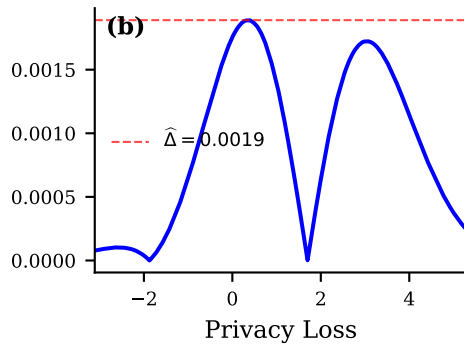
CDF Error
