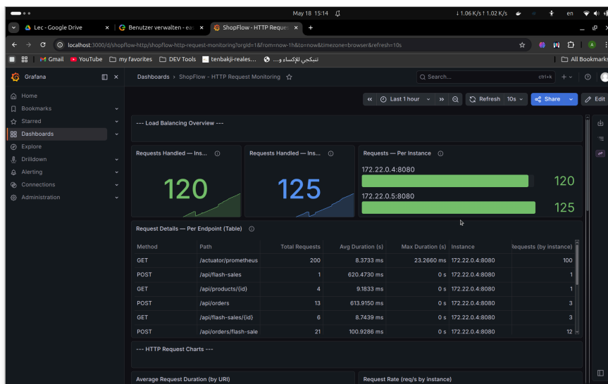
شكل 11: نظرة عامة على توزيع الأحمال — Instance 1: 120 طلب، Instance 2: 125 طلب (توزيع شبه متساوٍ عبر Round-Robin)
