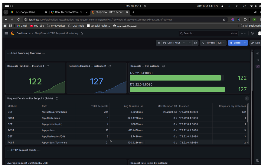
شكل 12: جدول تفصيلي بكل نقطة نهاية — المدة المتوسطة، المدة القصوى، النسبة المُعالجة، وعدد الطلبات لكل نسخة
