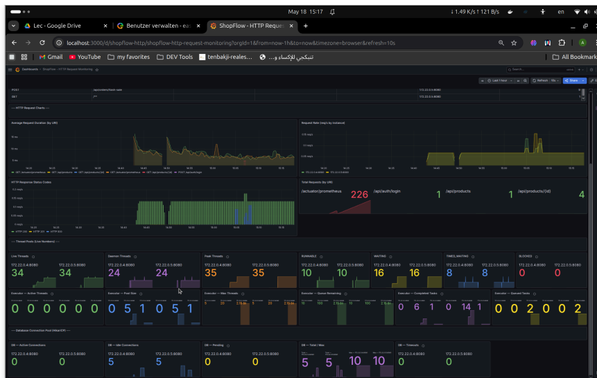
شكل 6: مقاييس مفصلة — رموز حالة (200, 201, 500) HTTP، إجمالي الطلبات لكل مسار، مع إحصائيات مجتمعات الخيوط (Executor Active/Pool Size/Max/Queue) وقاعدة البيانات (Active/Idle/Pending/Total Connections)
