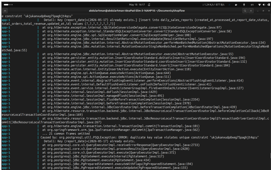
شكل 10: خطأ duplicate key — عندما تحاول كلتا النسختين إنشاء التقرير في الوقت ذاته، تفشل إحدهما بسبب القيد الفريد على report_date (سلوك متوقع ومحمي)
