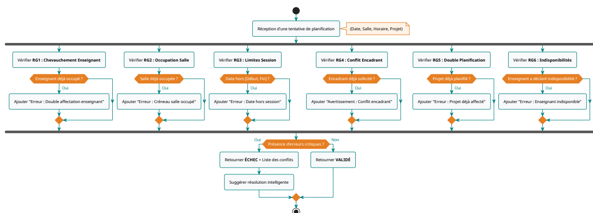
FIGURE 14 – Logique de validation des 6 règles de gestion (RG1-RG6)
