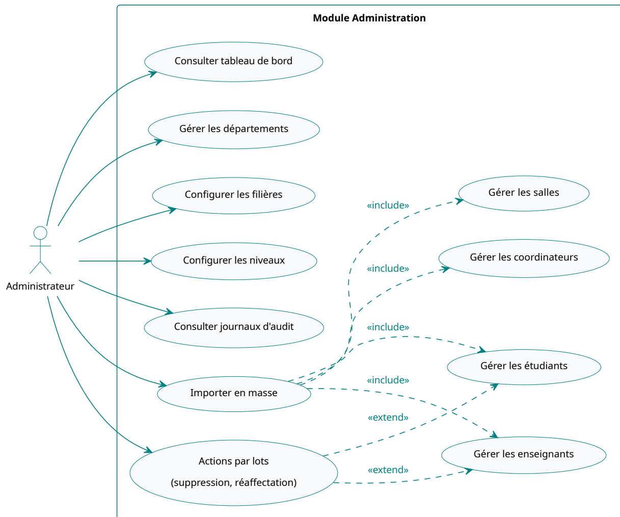
FIGURE 7 – Cas d'utilisation : Administration du système
