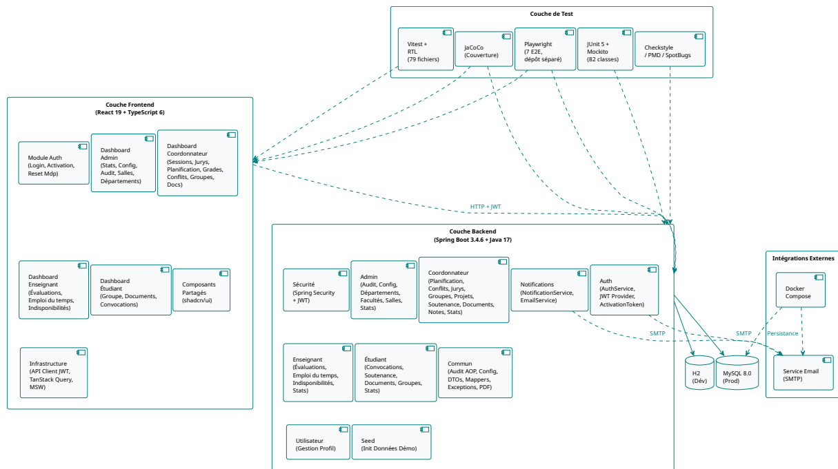
FIGURE 21 – Architecture en composants du système
