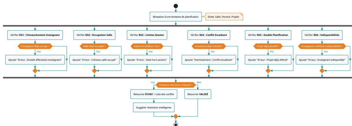
FIGURE 18 – Logique de validation des 6 règles de gestion (RG1-RG6)
