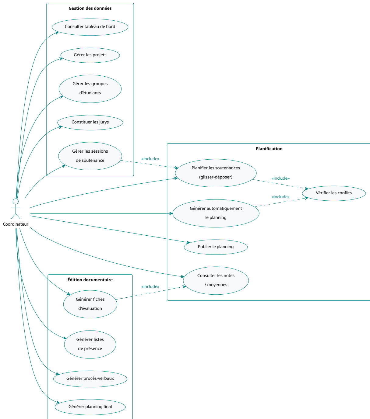
FIGURE 8 – Cas d'utilisation : Coordination et Defense Designer
