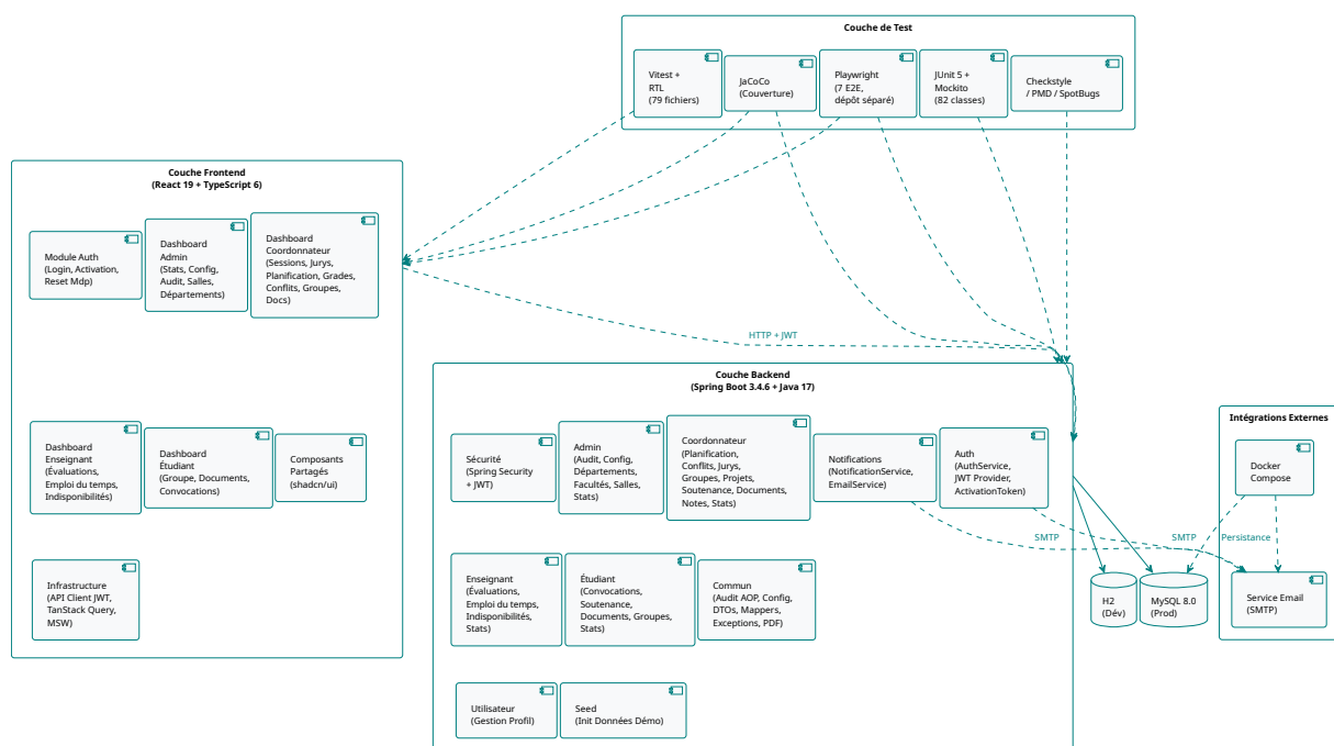
FIGURE 16 – Architecture en composants du système
