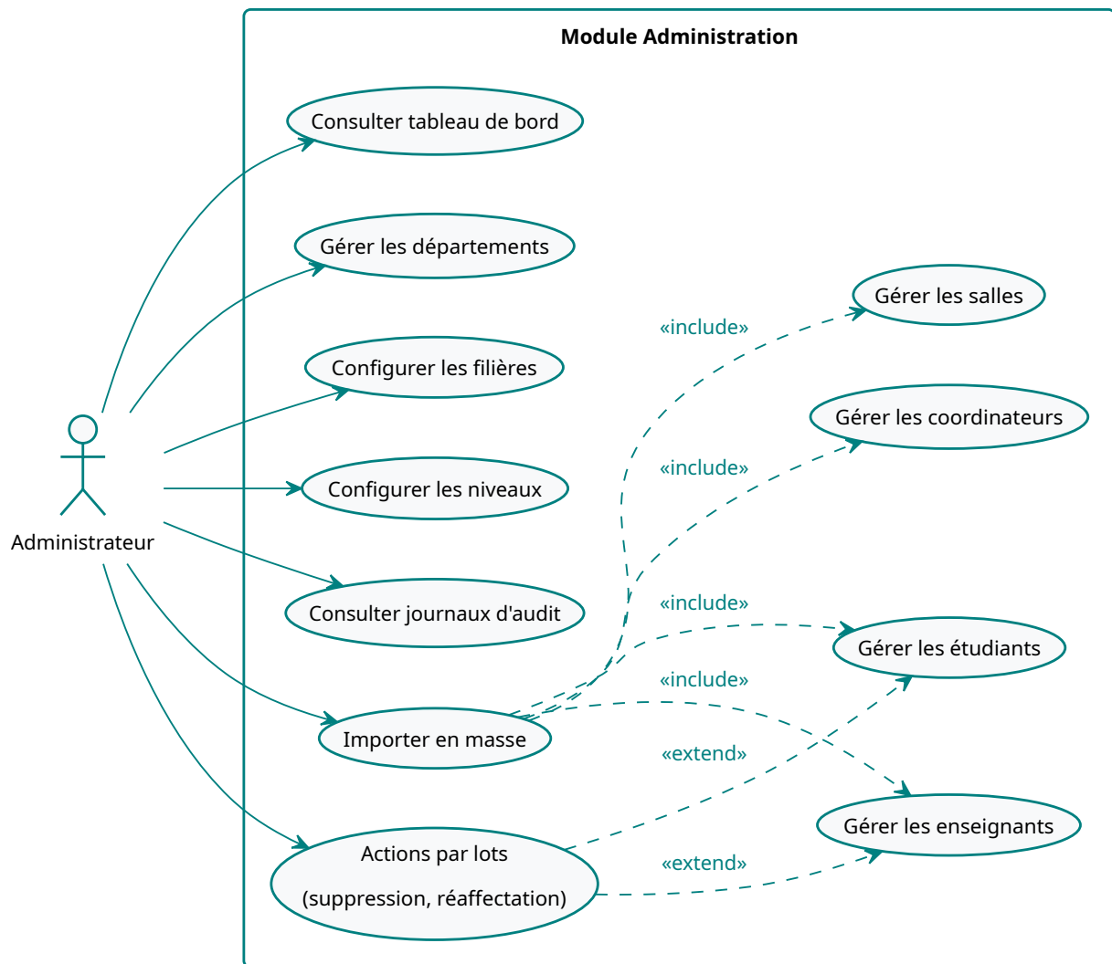
FIGURE 7 – Cas d'utilisation : Administration du système
