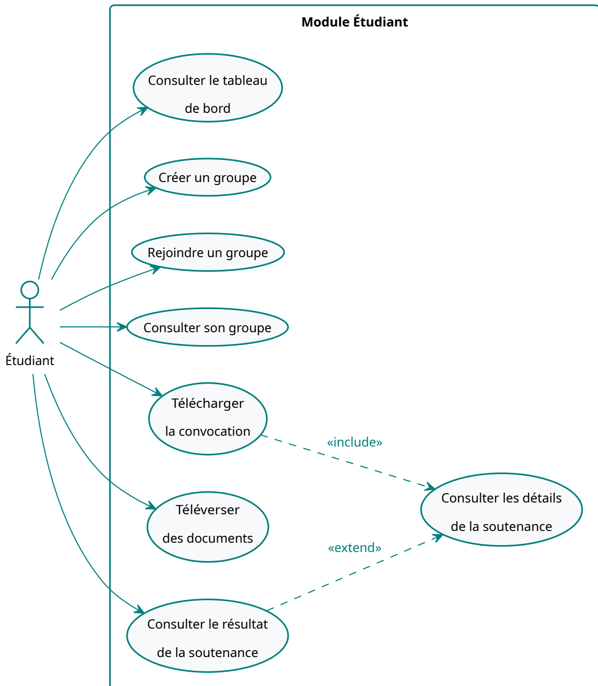
FIGURE 10 – Cas d'utilisation : Étudiant
