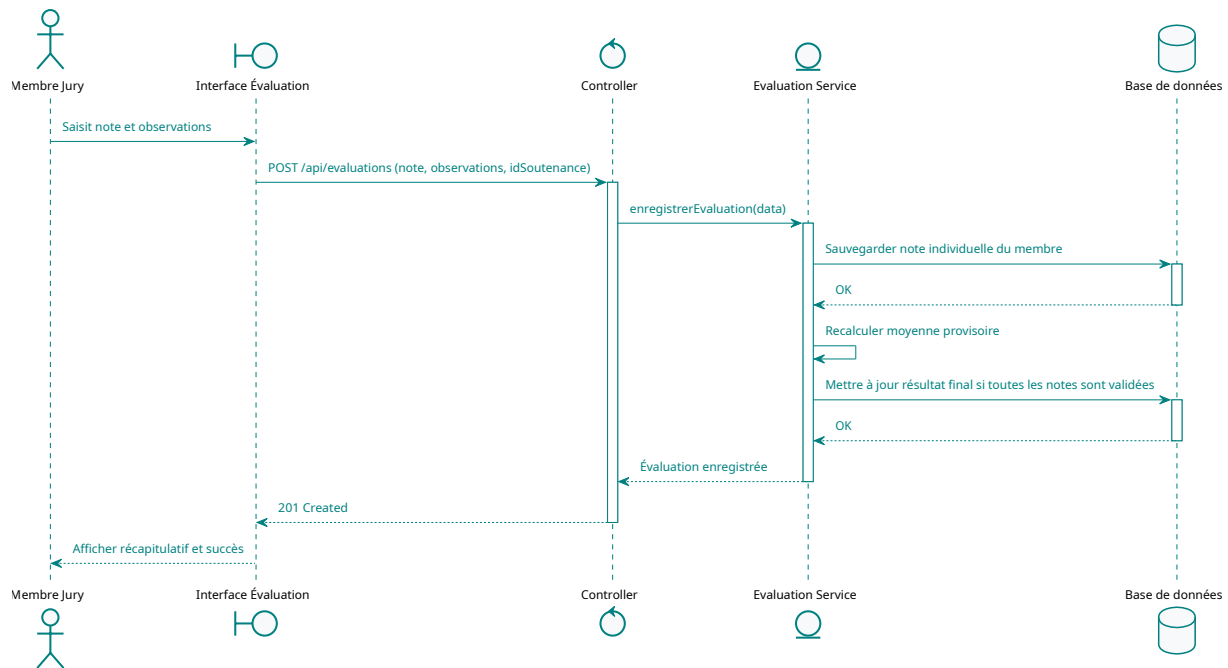
FIGURE 17 – Séquence de soumission d'une évaluation
