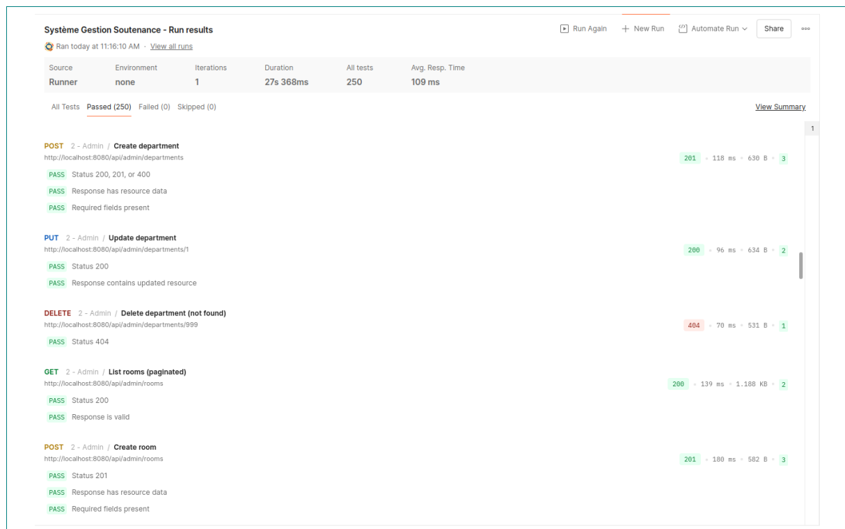
FIGURE 40 – Collection Postman – 250 assertions passant avec succès
