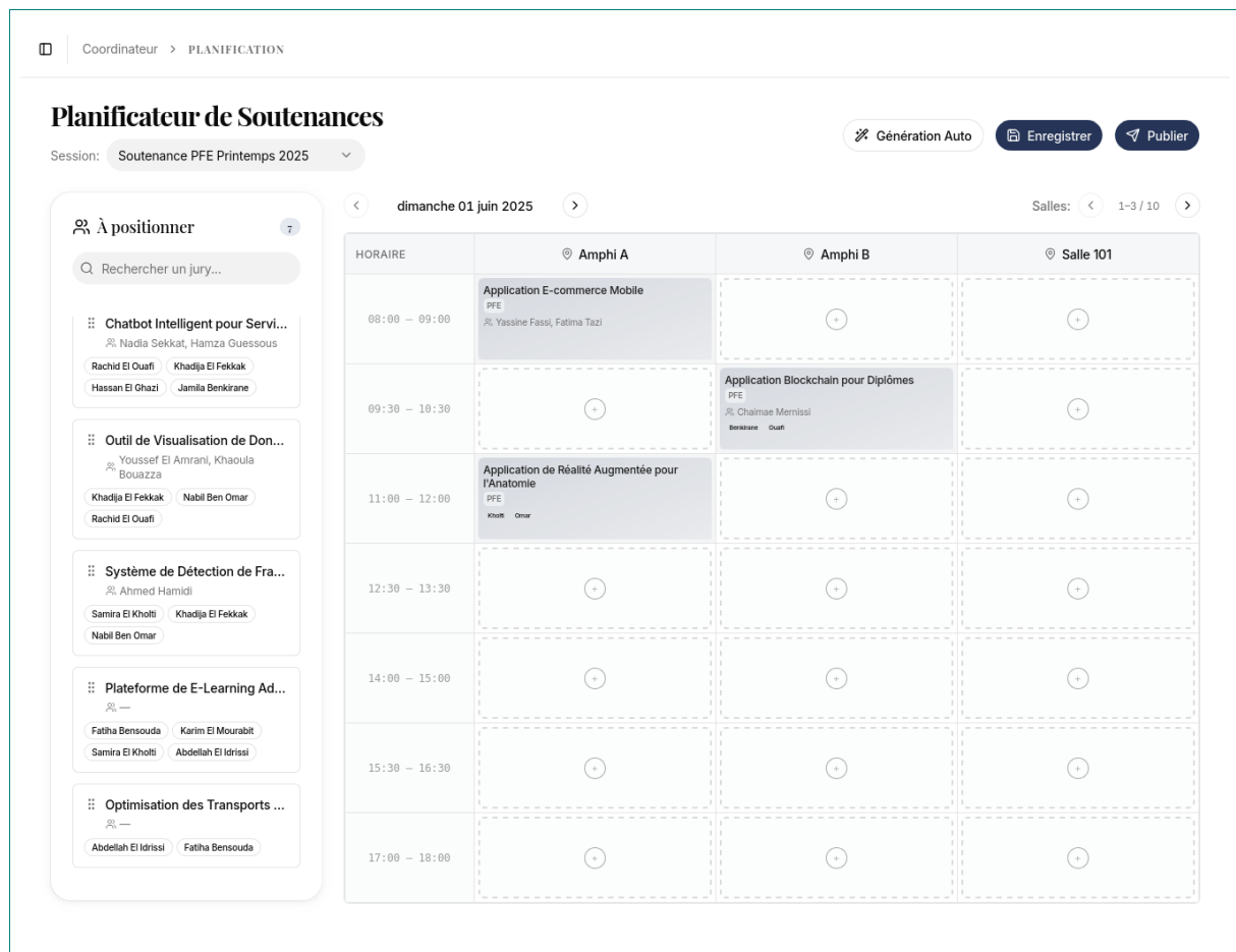
FIGURE 30 – Defense Designer – interface de planification interactive par glisser-déposer
