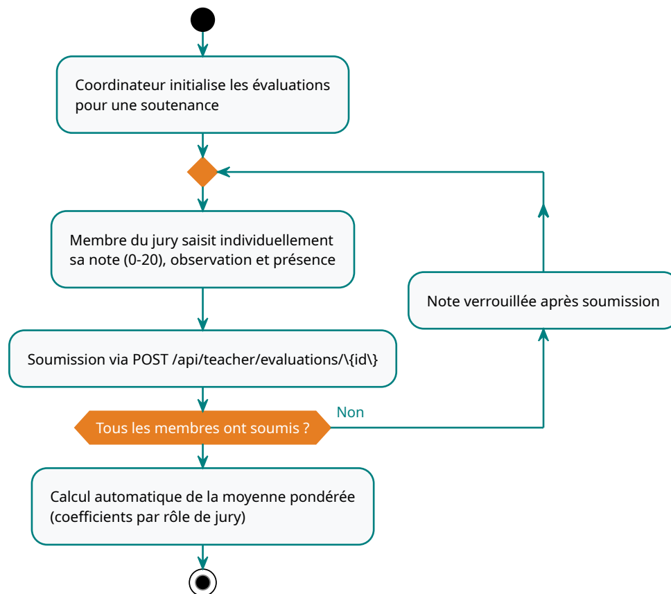
FIGURE 20 – Processus d'évaluation et de notation d'une soutenance
