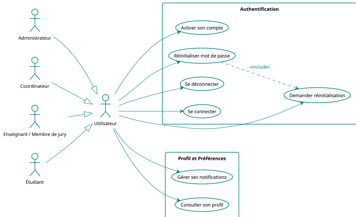
FIGURE 6 – Hiérarchie générale des acteurs
