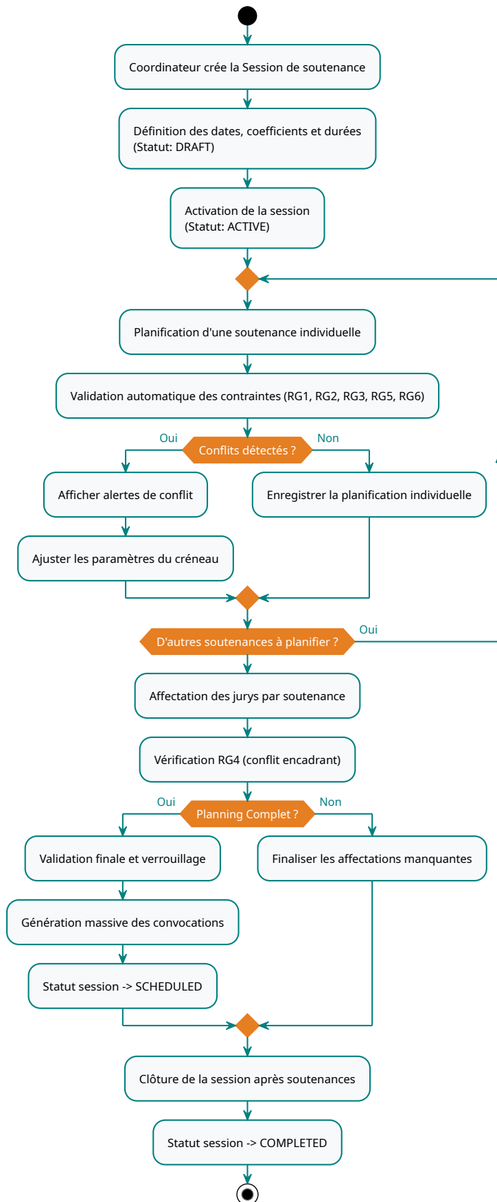
FIGURE 19 – Diagramme d'activité du processus de planification
