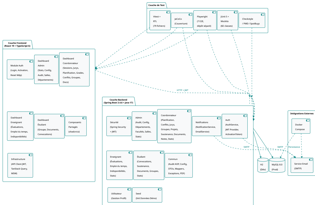
FIGURE 21 – Architecture en composants du système
