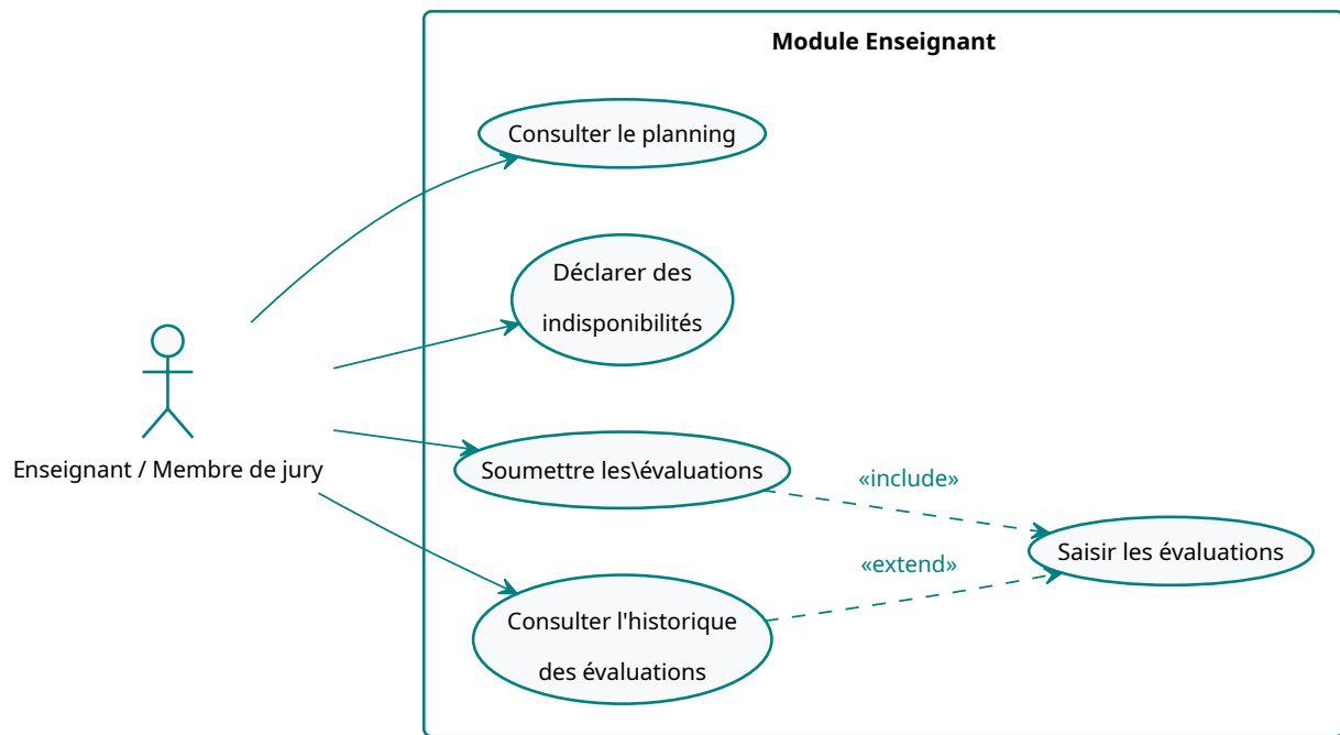
FIGURE 9 – Cas d'utilisation : Enseignant / Membre de jury
