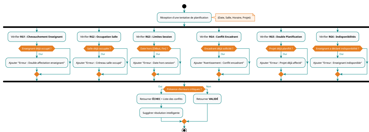
FIGURE 18 – Logique de validation des 6 règles de gestion (RG1-RG6)
