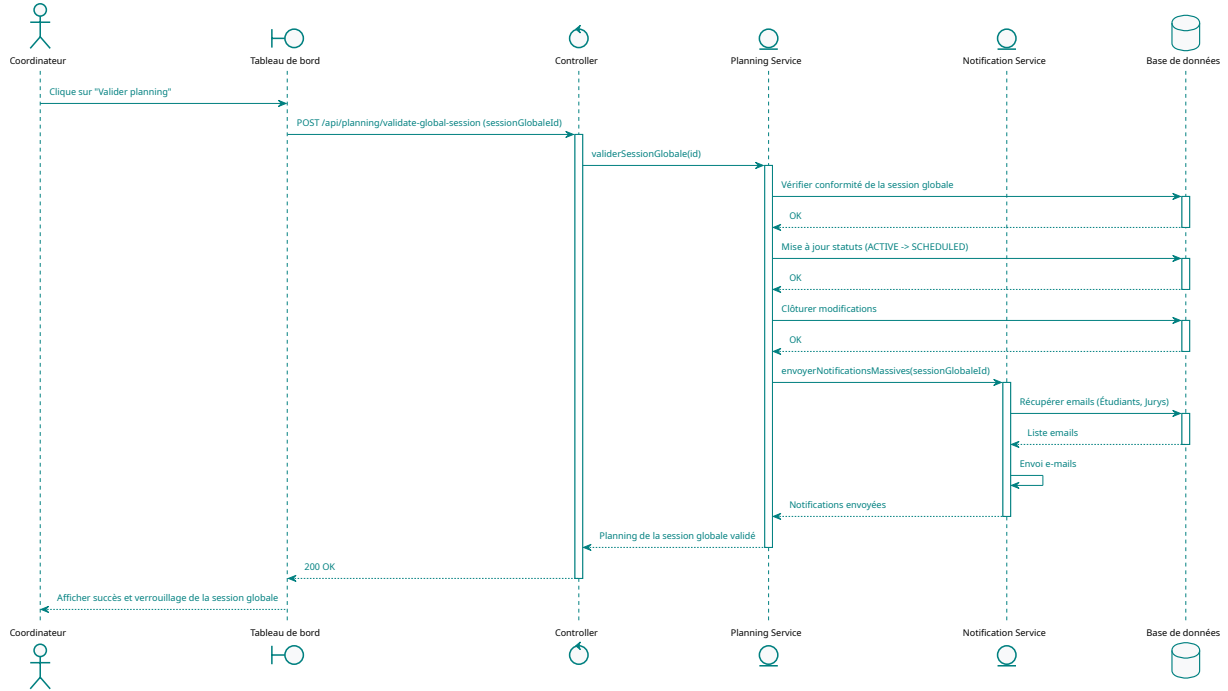
FIGURE 14 – Séquence de validation globale et verrouillage de la session
