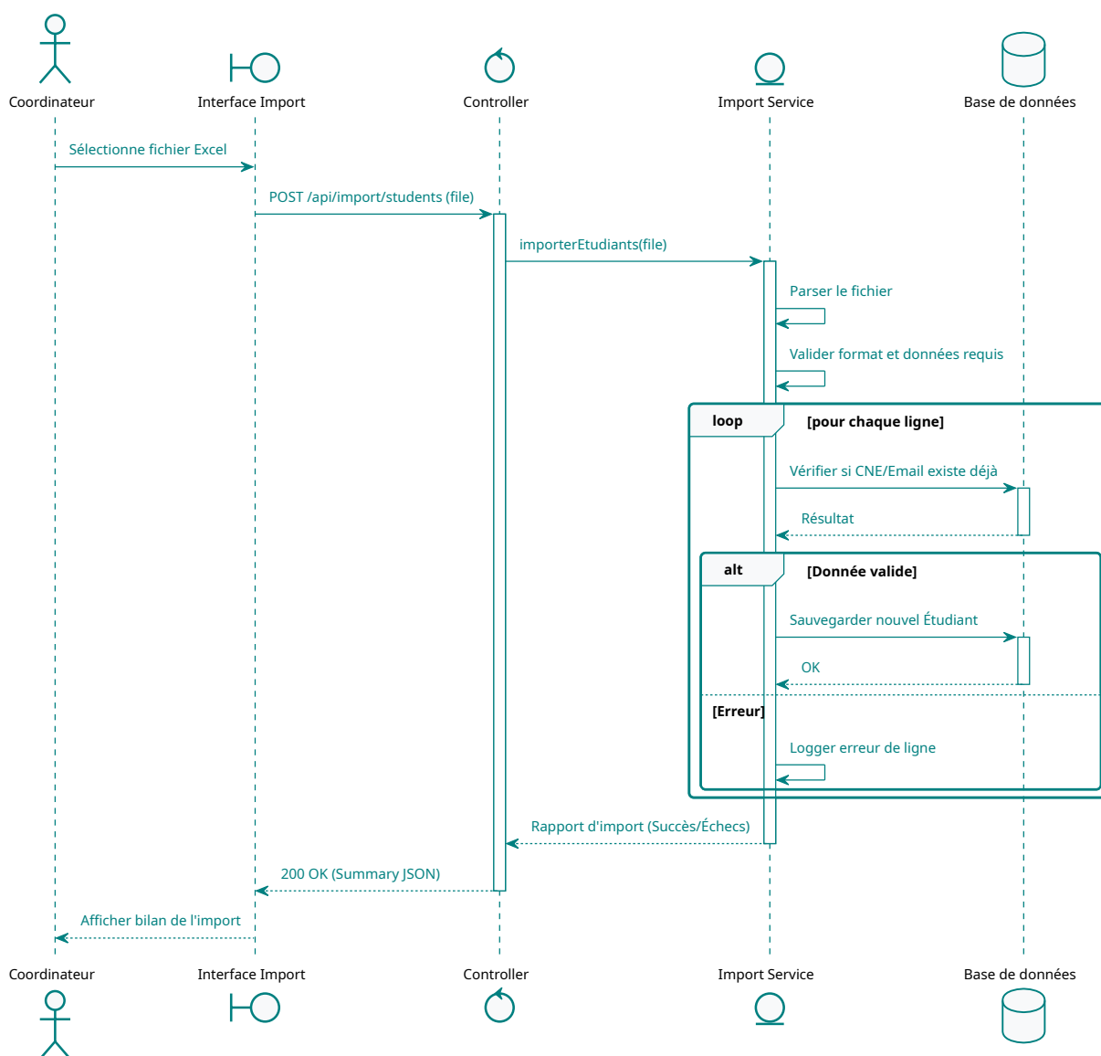
FIGURE 5 – Séquence d'importation massive des données depuis un fichier Excel
