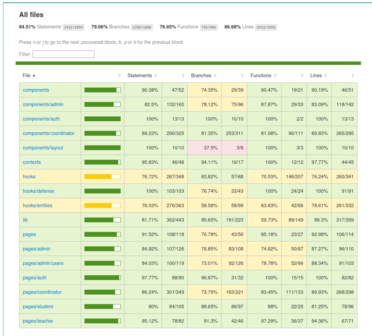
FIGURE 39 – Rapport de couverture de code frontend (Vitest + v8)
