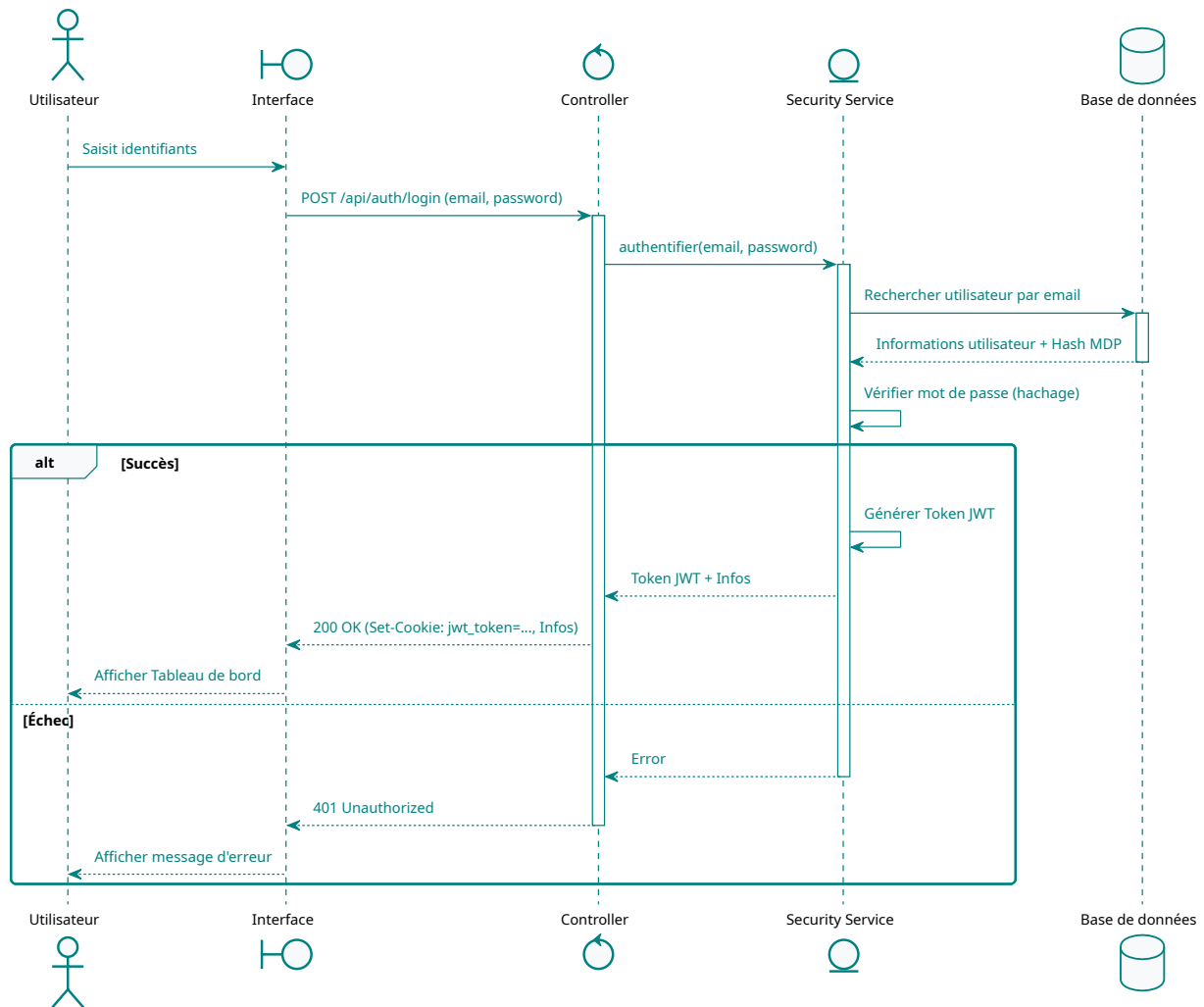
FIGURE 16 – Séquence d'authentification via JWT
