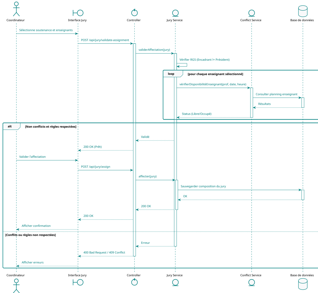
FIGURE 12 – Séquence d'affectation et de validation des membres du jury
