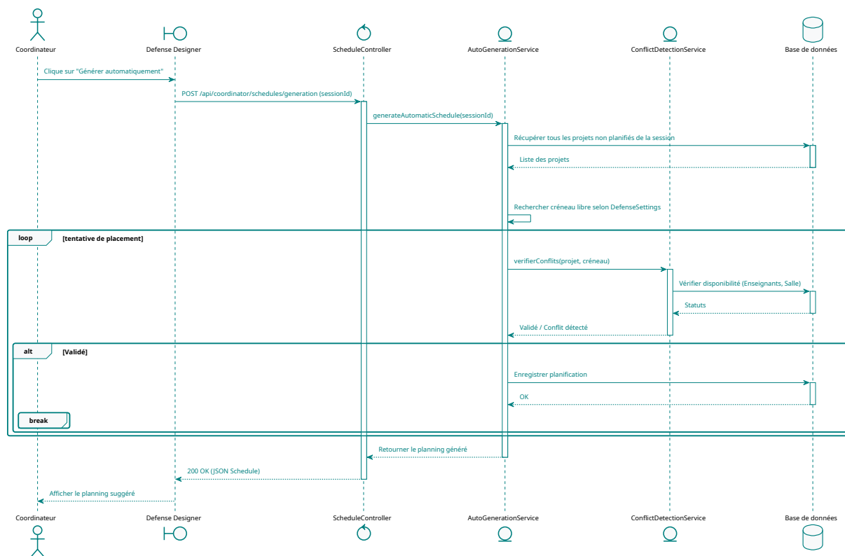
FIGURE 15 – Séquence de l’algorithme d’auto-génération du planning
