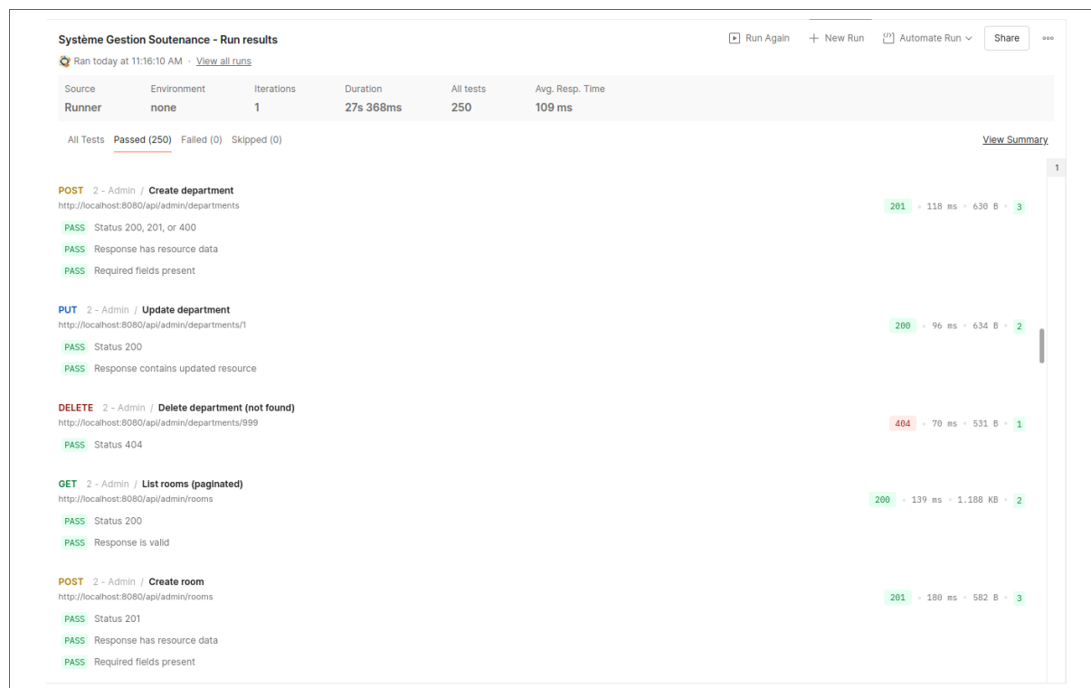
FIGURE 38 – Collection Postman – 250 assertions passant avec succès
