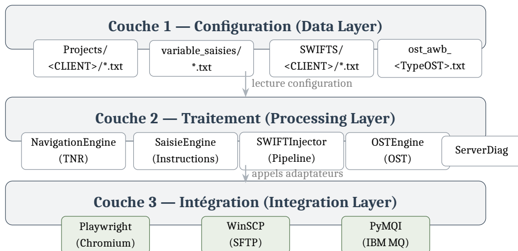
Figure 3.1 – Architecture à trois couches du framework d'automatisation
