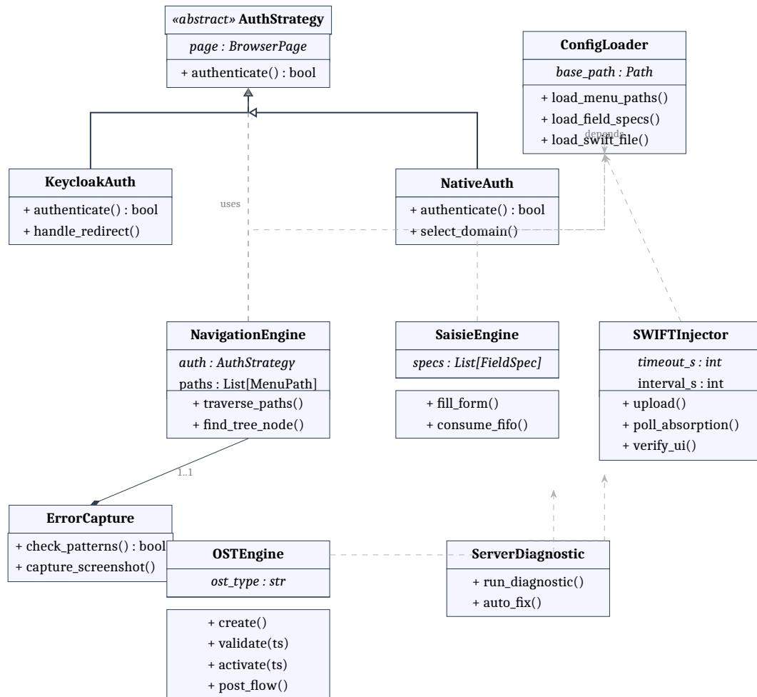
Figure 3.3 – Diagramme de classes — Structure conceptuelle du framework
