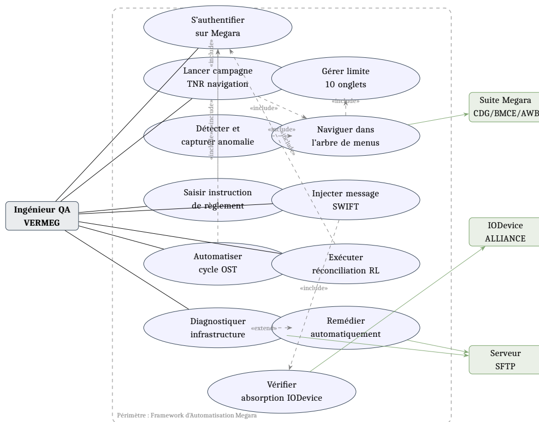
Figure 3.2 – Diagramme de cas d'utilisation — Framework d'automatisation Megara
