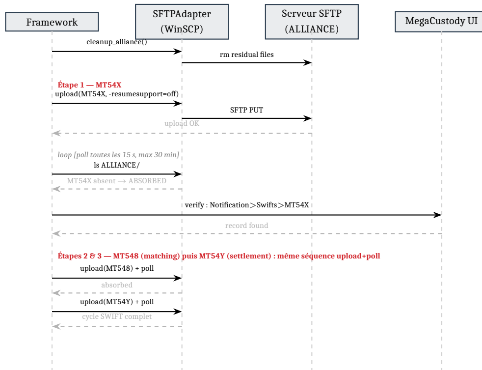
Figure 3.5 – Diagramme de séquence — Pipeline d’injection SWIFT end-to-end
