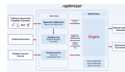
Optimizer
