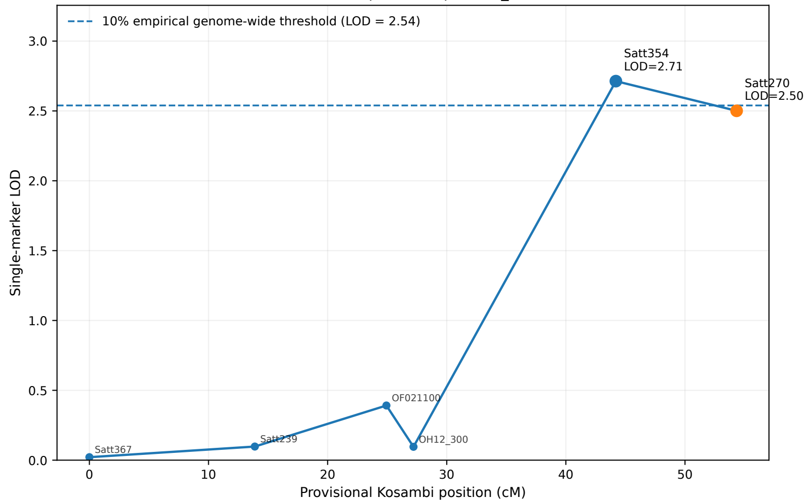
SCN F13 QTL profile on pLG01b_Gm20
