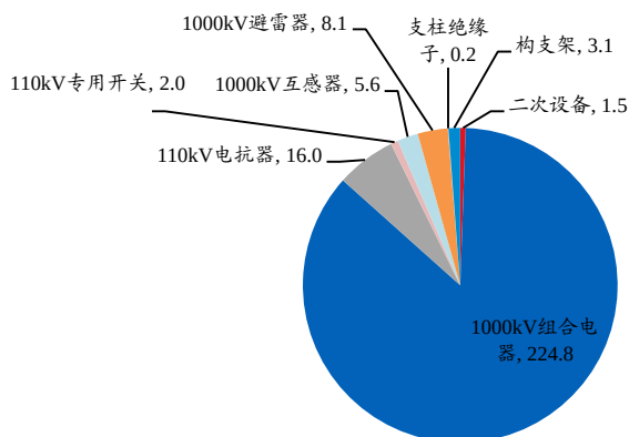
图表 3 成都东 1000kV 变电站阿坝 1000 千伏间隔扩建工程设备采购情况（百万元）
